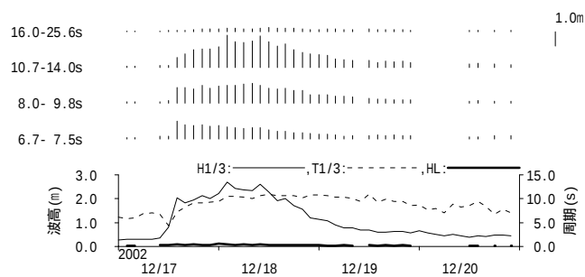
付図 - B.1.28 釜石 周期帯別波浪特性の経時変化(高波期間中)
