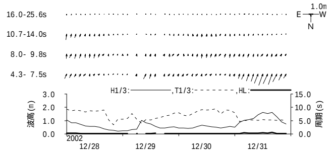
付図 - B.1.8 富山 周期帯別波浪特性の経時変化(高波期間中)
