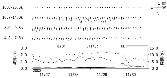
付図 - B.1.8 富山 周期帯別波浪特性の経時変化(高波期間中)
