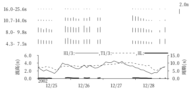
付図-B.1.11 金沢 周期帯別波浪特性の経時変化(高波期間中)
