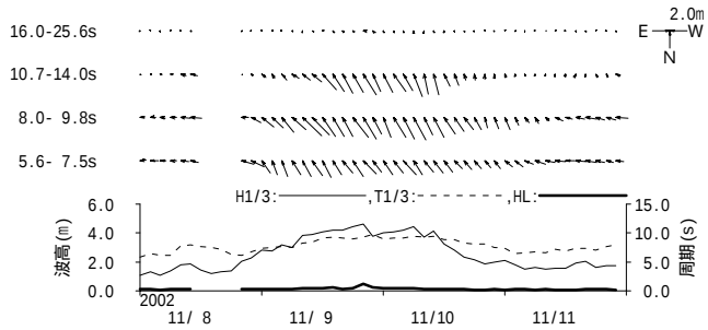
付図 - B.1.10 輪島 周期帯別波浪特性の経時変化(高波期間中)
