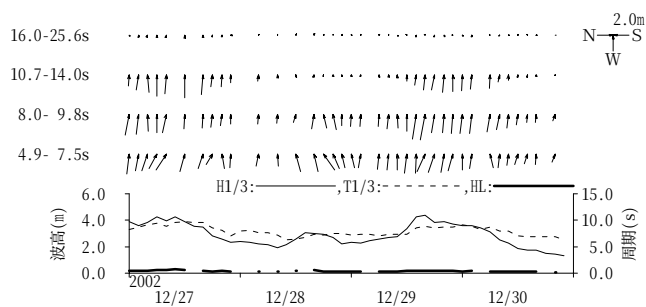
付図-B.1.4 秋田 周期帯別波浪特性の経時変化(高波期間中)
