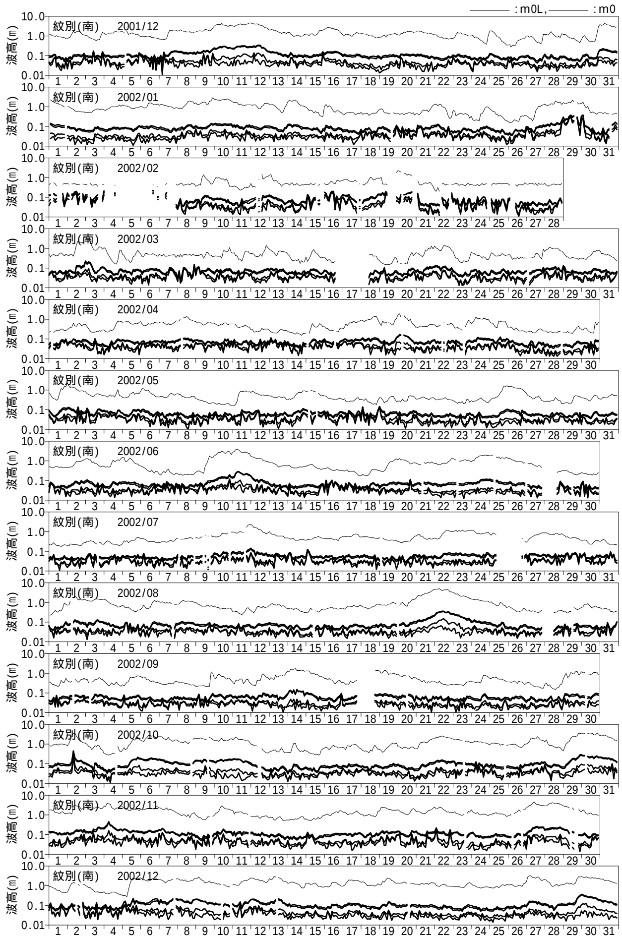
付図 - A.2.22 長周期波高の経時変化図（紋別(南)）
