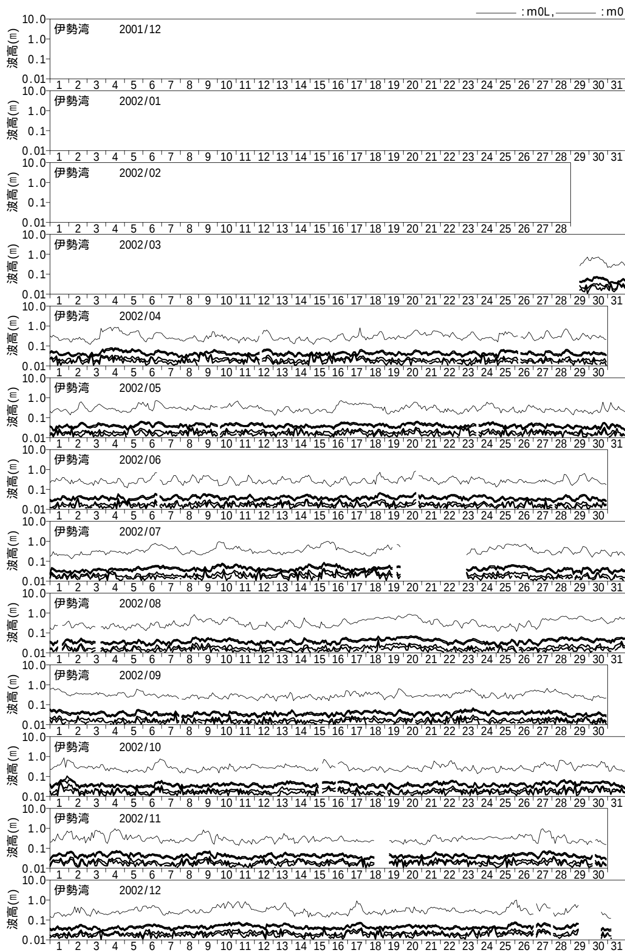
付図 - A.2.41 長周期波高の経時変化図 (伊勢湾)
