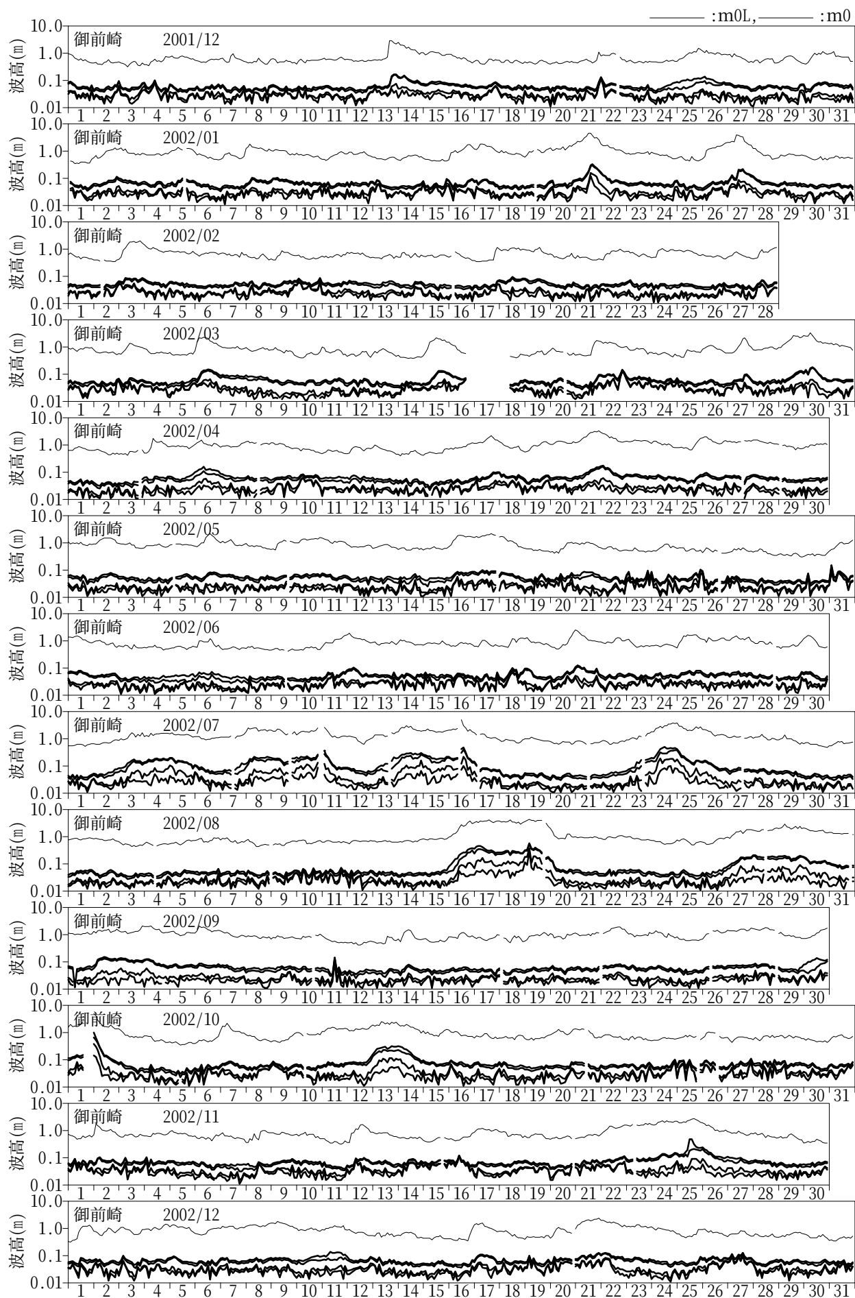
付図-A.2.40 長周期波高の経時変化図（御前崎）
