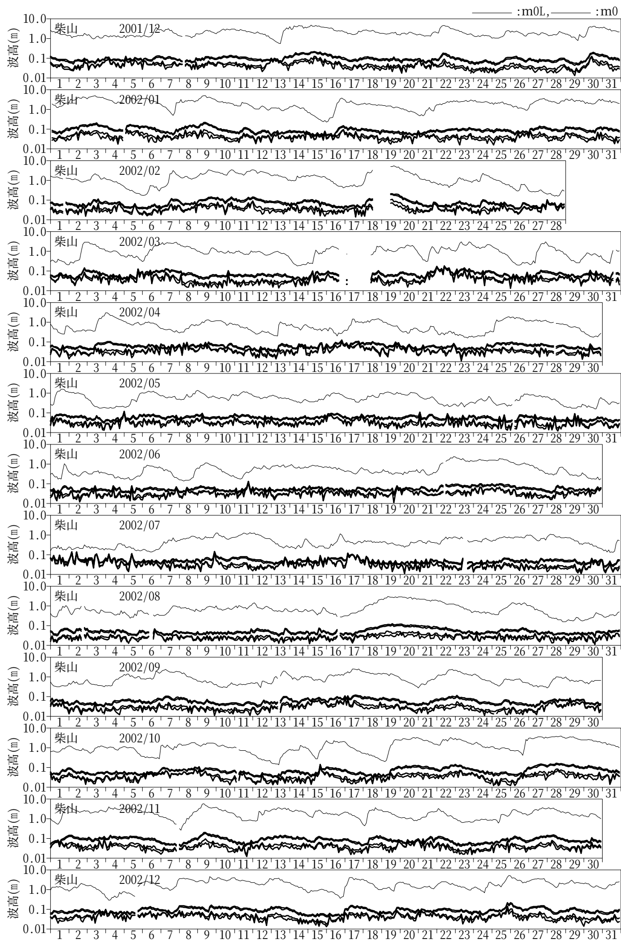
付図-A.2.12 長周期波高の経時変化図（柴山）
