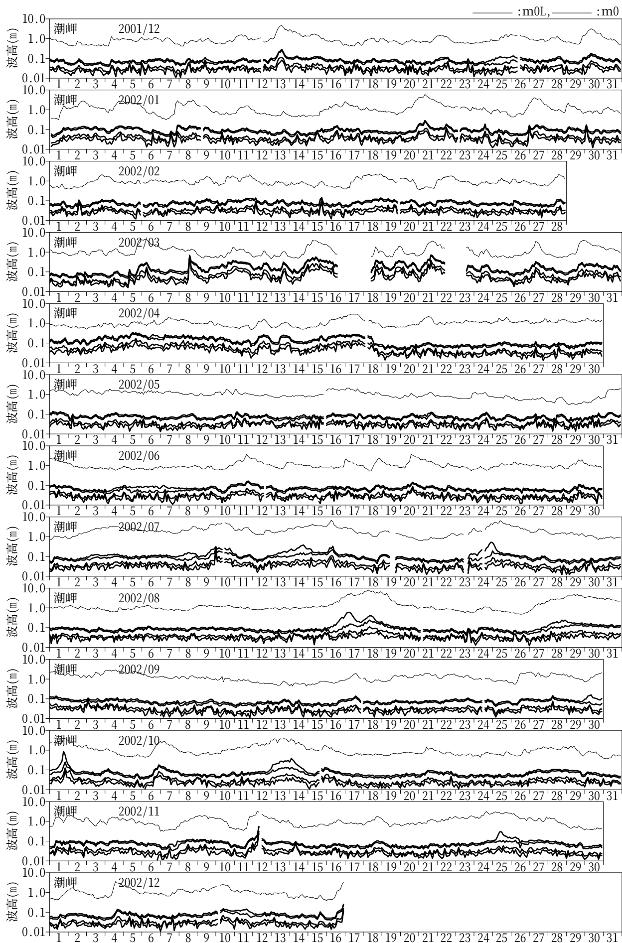
付図-A.2.42 長周期波高の経時変化図（潮岬）
