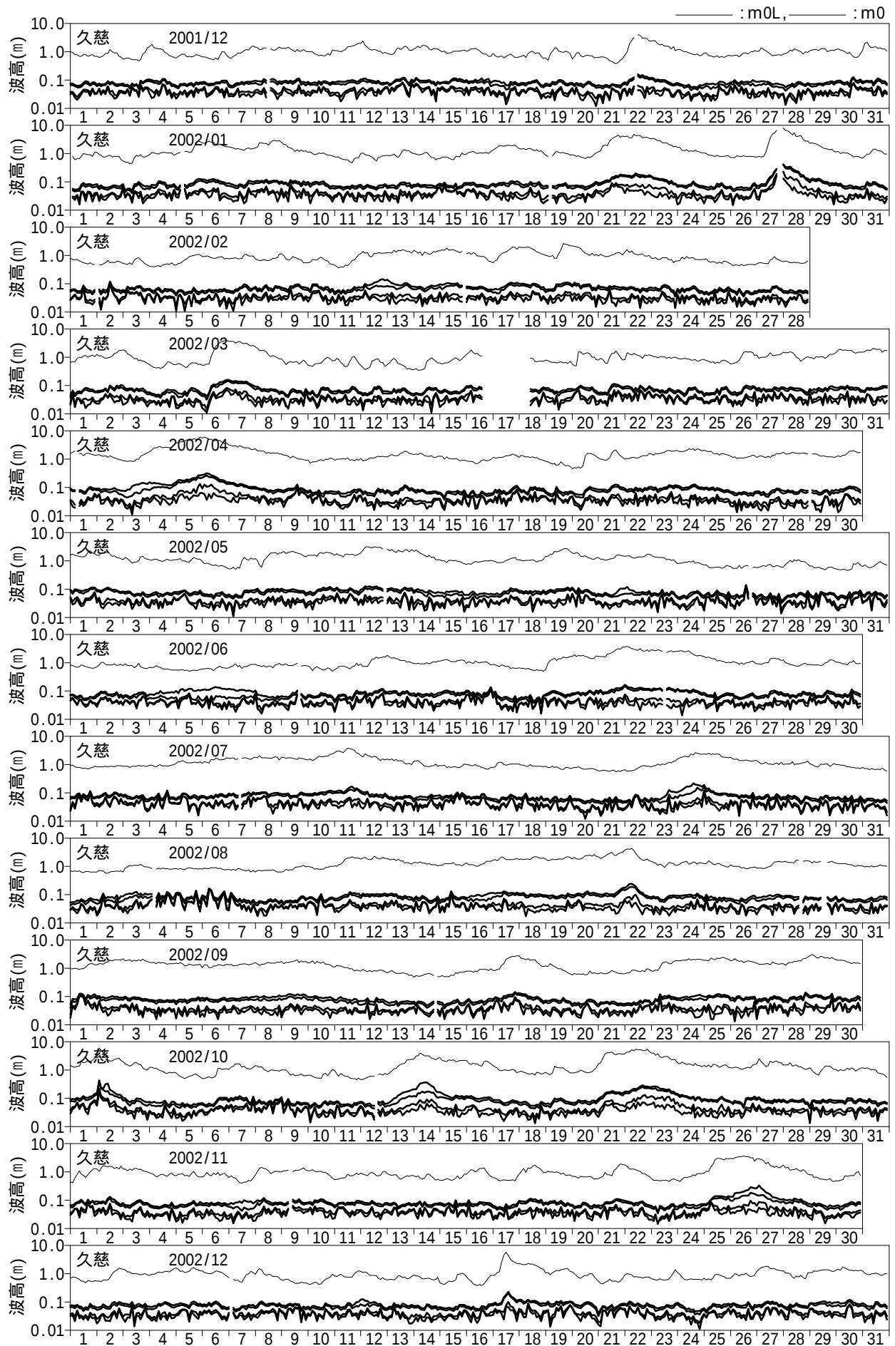
付図 - A.2.27 長周期波高の経時変化図 (久慈)
