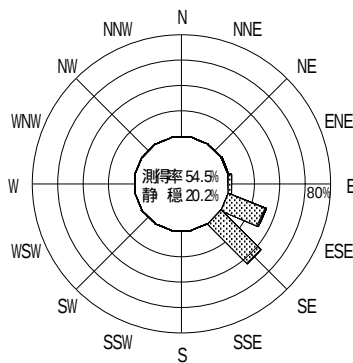
図 - 8.44 小松島 波高・波向別出現頻度図
