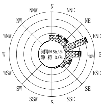
2001年12月～2002年 2月 (冬)
