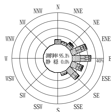
2002年 1月～2002年12月 (年)
