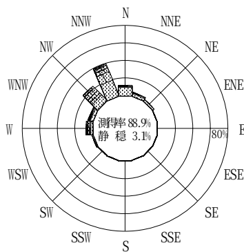
図-8.7 直江津 波高・波向別出現頻度図
