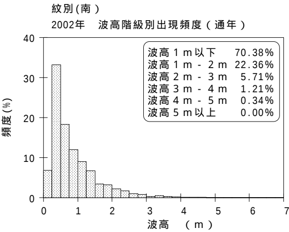
図 - 7.22 紋別(南) 波候特性図
