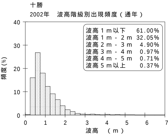
図 - 7.23 十勝 波候特性図
