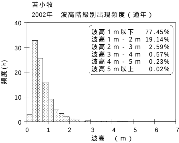
図 - 7.24 苫小牧 波候特性図
