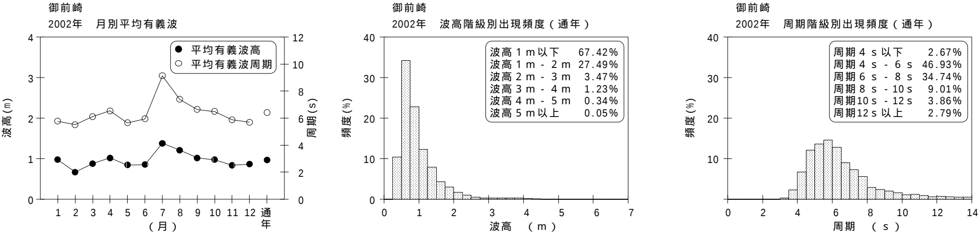
図 - 7.40 御前崎 波候特性図
