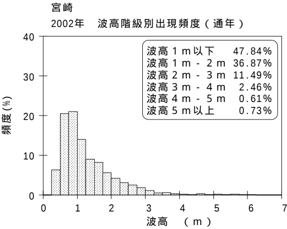
図 - 7.50 宮崎 波候特性図
