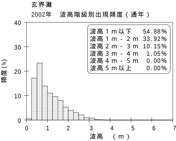
図 - 7.18 玄界灘 波候特性図
