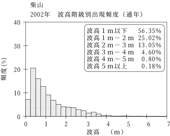
図-7.12 柴山 波候特性図
