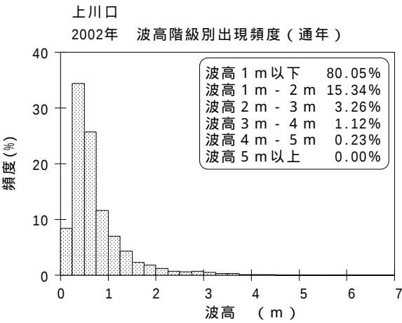
図 - 7.47 上川口 波候特性図
