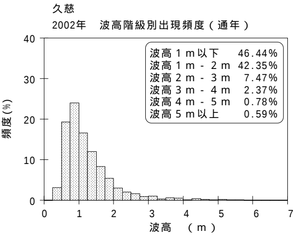
図 - 7.27 久慈 波候特性図
