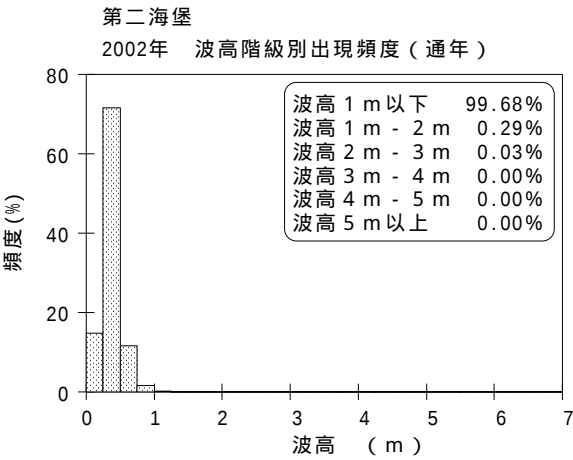
図 - 7.35 第二海堡 波候特性図
