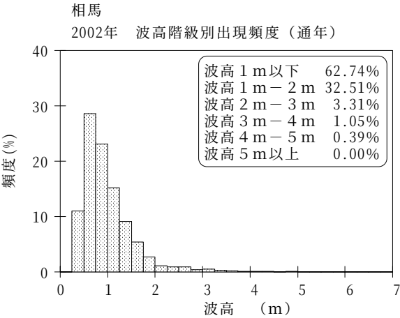
図－7.31 相馬 波候特性図
