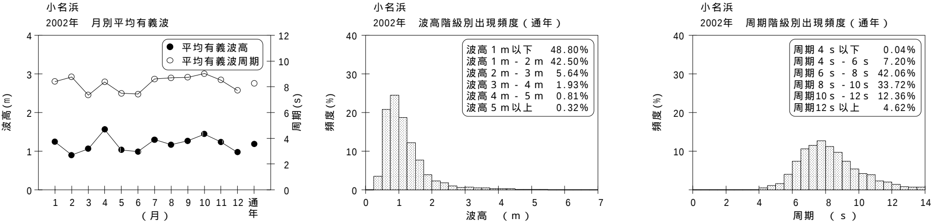
図 - 7.32 小名浜 波候特性図
