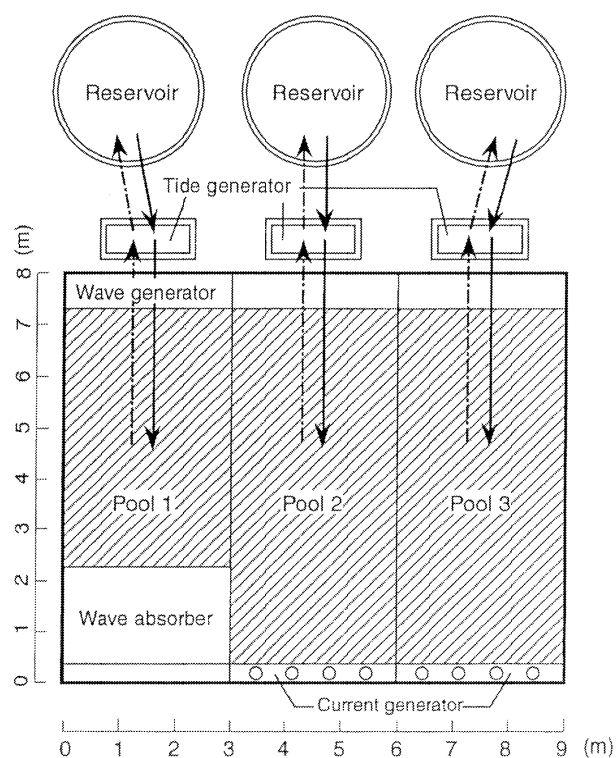
図-3 実験水槽の平面図と実験海水のフロー、実線が上げ潮、破線が下げ潮を示す。
