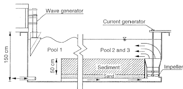
図-4 実験水槽の断面図
