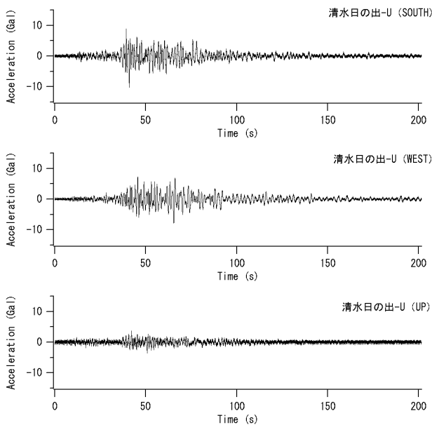
図-30 清水日の出-Uにおけるオリジナル加速度波形
