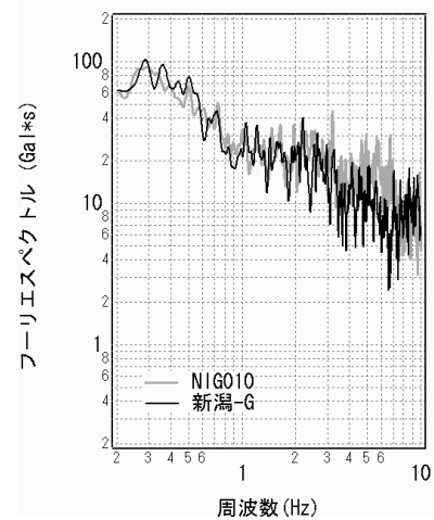
図-31 新潟-Gにおけるフーリエスペクトル(NIG010におけるフーリエスペクトルを併記)
