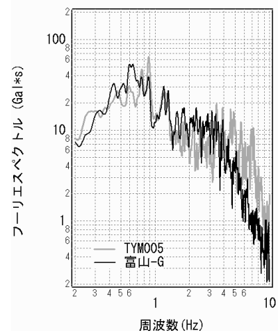
図-32 富山-Gにおけるフーリエスペクトル(TYM005におけるフーリエスペクトルを併記)
