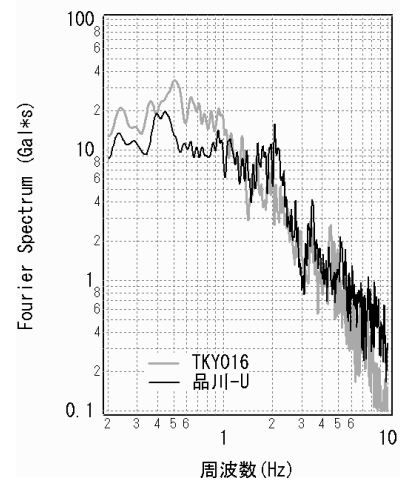
図-33 品川-Uにおけるフーリエスペクトル(TKY016におけるフーリエスペクトルを併記)
