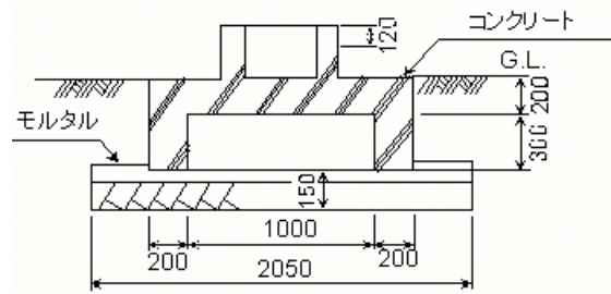
A-A断面
