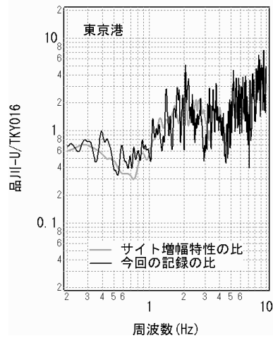
図-35 中小地震記録によるサイト増幅特性 3) の比と今回の記録のスペクトル比 (品川-U/TKY016)
