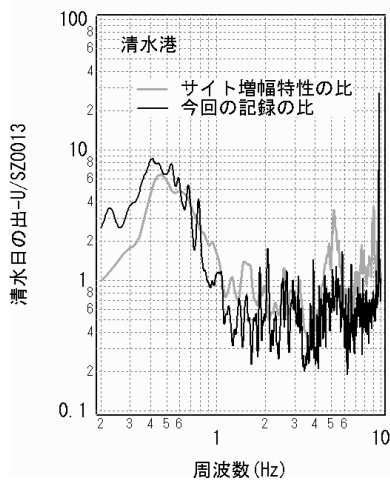
図-36 中小地震記録によるサイト増幅特性 3) の比と今回の記録のスペクトル比 (清水日の出-U/SZ0013)
