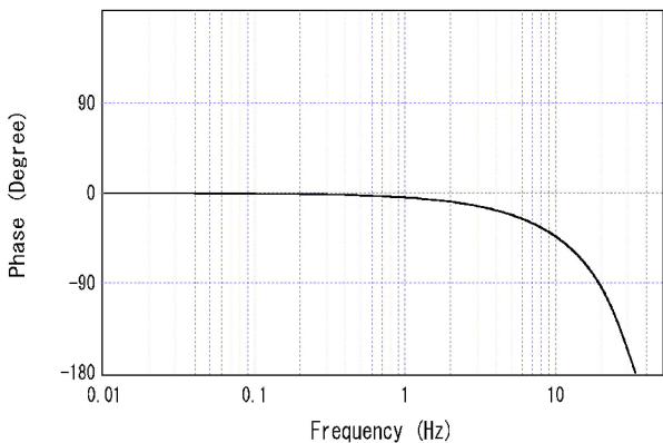
図-17 SMAC-MDU 型強震計の周波数特性
