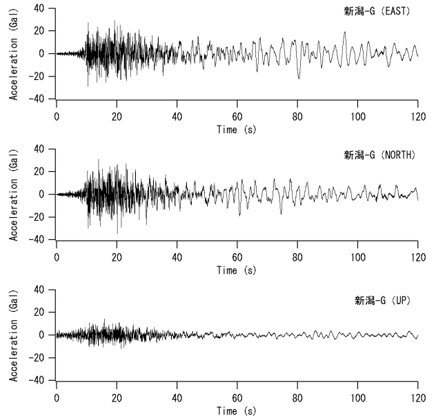
図-27 新潟-G におけるオリジナル加速度波形
