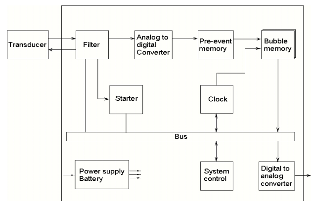
図-11 ERS-F 型強震計のブロックダイアグラム
