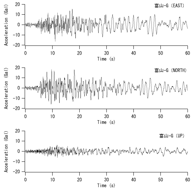
図-28 富山-G におけるオリジナル加速度波形
