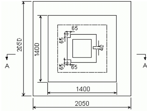
平面図 単位：mm
