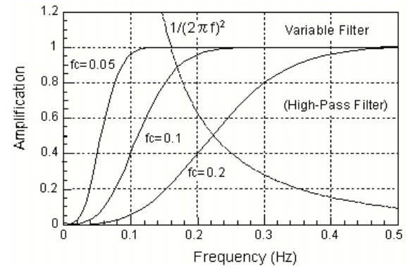
図-23 パラメタ付きフィルタと二回積分
