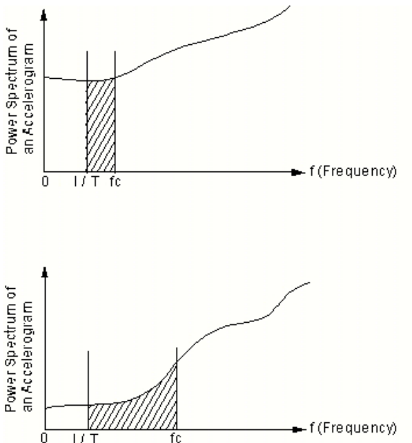
図-25 f_c の決定手順
