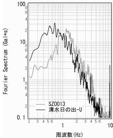
図-34 清水日の出-U におけるフーリエスペクトル (SZ0013 におけるフーリエスペクトルを併記)
