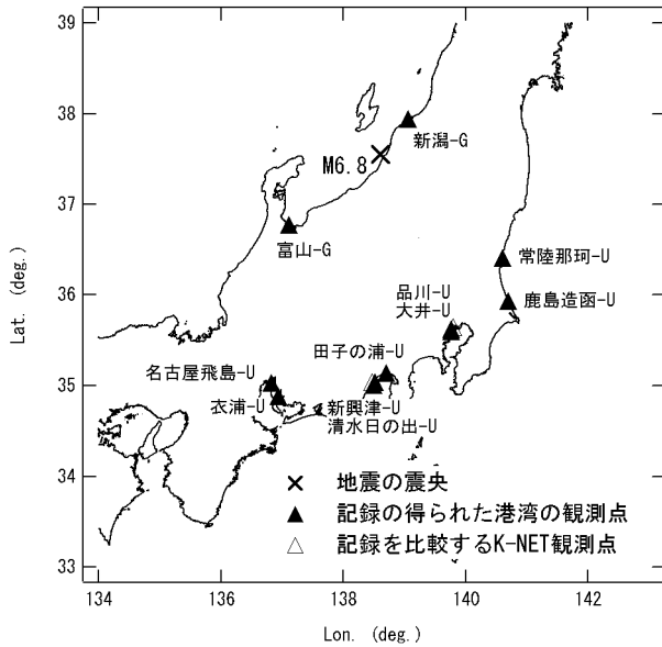
図-26 2007年新潟県中越沖地震 (M6.8) の震央 (×) と記録の得られた港湾の位置 (▲)
