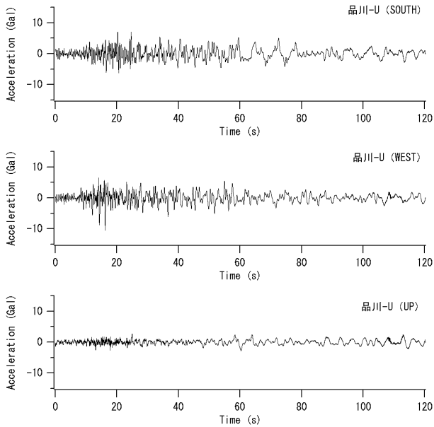
図-29 品川-Uにおけるオリジナル加速度波形
