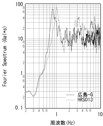
図-34 広島-G におけるフーリエスペクトル (HRS013 におけるフーリエスペクトルを併記)
