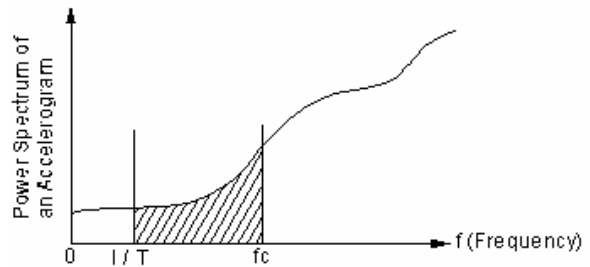
図-25 f_c の決定手順
