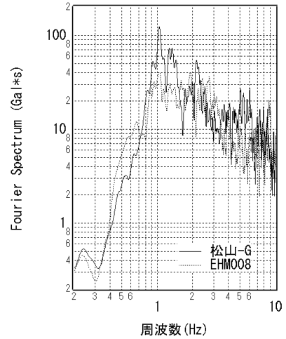
図-36 境港-G におけるフーリエスペクトル (SMN001 におけるフーリエスペクトルを併記)
