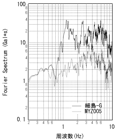
図-33 細島-G におけるフーリエスペクトル (MYZ005 におけるフーリエスペクトルを併記)
