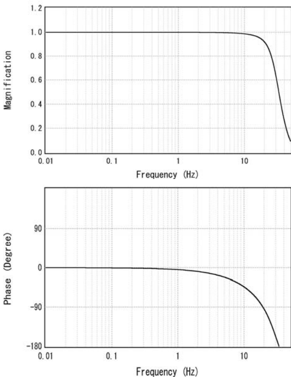
図-17 SMAC-MDU 型強震計の周波数特性
