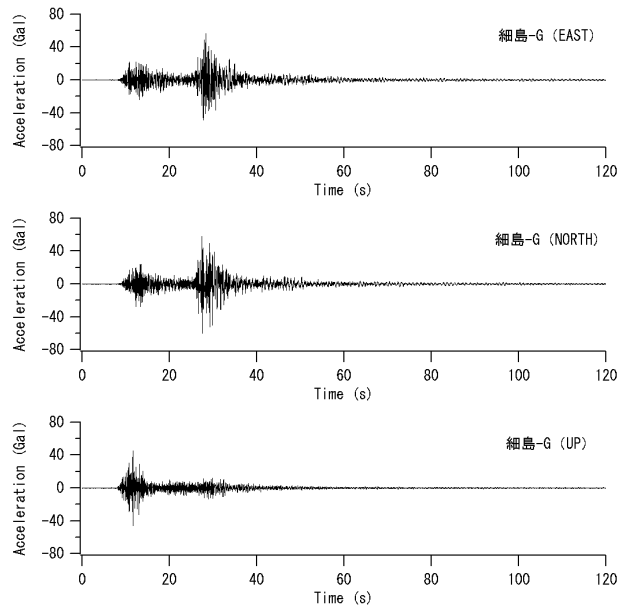
図-29 細島-Gにおけるオリジナル加速度波形
