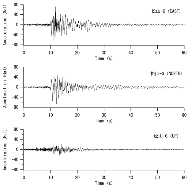
図-31 松山-Gにおけるオリジナル加速度波形
