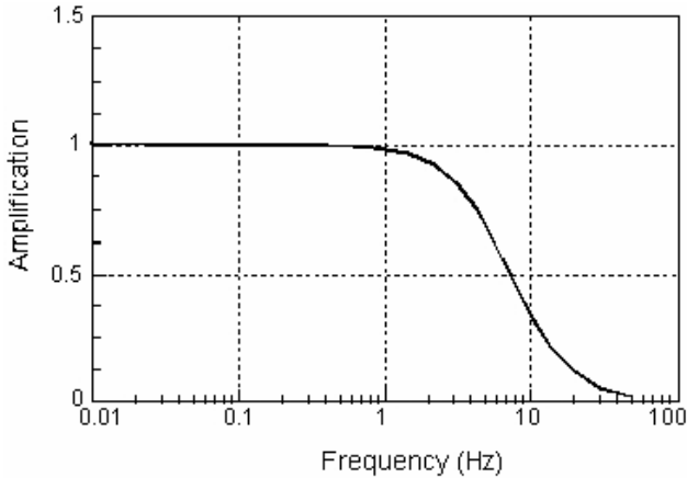
図-21 SMAC-B2 相当フィルタ
