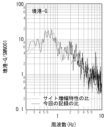
図-39 中小地震記録によるサイト増幅特性 65) の比と今回の記録のスペクトル比 (松山-G/EHM008)
