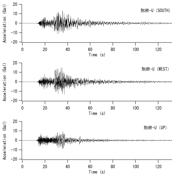
図-27 別府-Uにおけるオリジナル加速度波形
