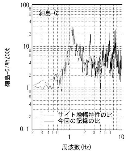
図-37 中小地震記録によるサイト増幅特性 65) の比と今回の記録のスペクトル比 (細島-G/MYZ005)
