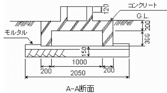
図-18 強震計基礎の一例
