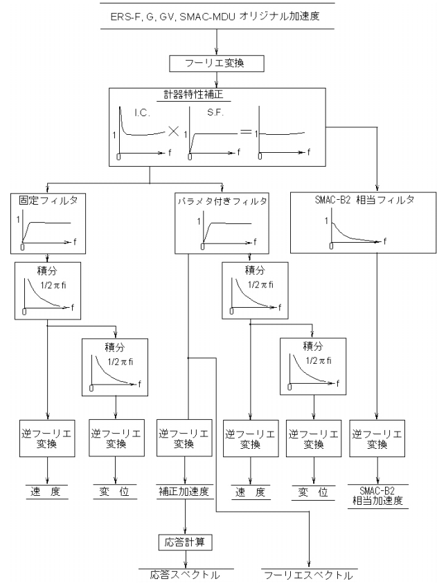
図-20 補正と積分の手順
