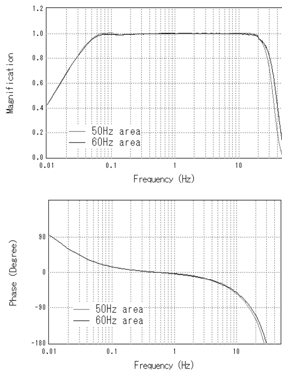
図-14 ERS-GV 型強震計の周波数特性
