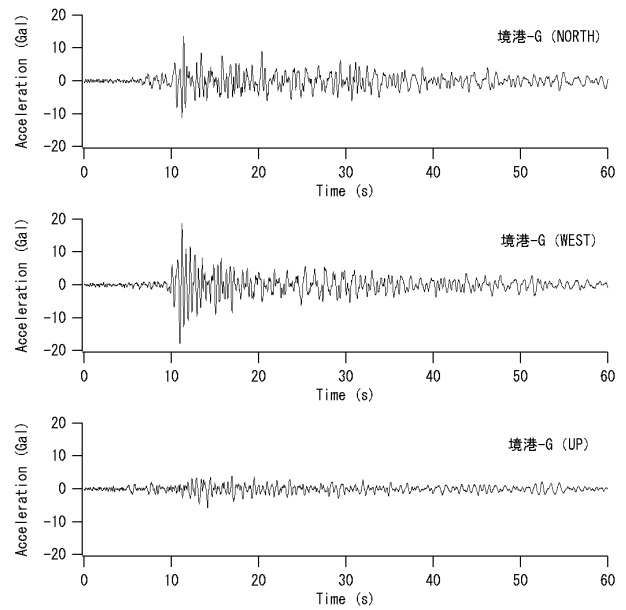
図-32 境港-Gにおけるオリジナル加速度波形
