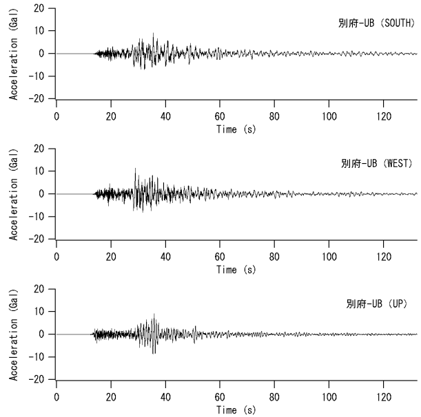
図-28 別府-UBにおけるオリジナル加速度波形
