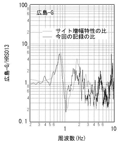
図-38 中小地震記録によるサイト増幅特性 65) の比と今回の記録のスペクトル比 (広島-G/HRS013)
