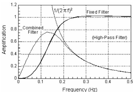
図-22 固定フィルタと二回積分の合成
