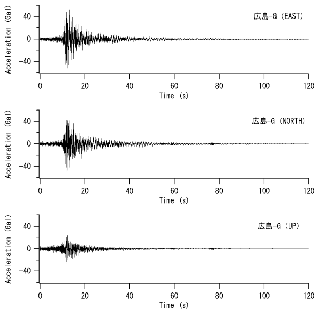
図-30 広島-Gにおけるオリジナル加速度波形
