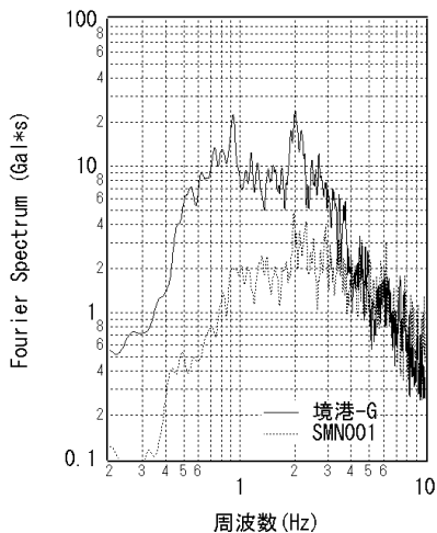
図-35 松山-G におけるフーリエスペクトル (EHM008 におけるフーリエスペクトルを併記)
