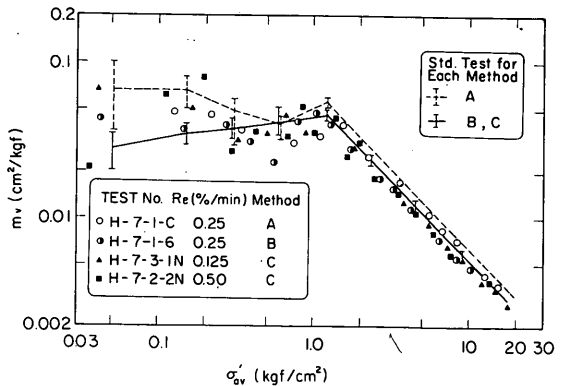
図-8.18 a m_v \sim \sigma'_{ov} 関係に及ぼす試験法の影響 (Mix.No.7 試料)
