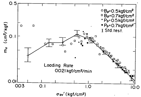
図 - 4.6 c 予圧密とバックプレッシャーの影響 (CLR-Test, 本牧再圧密試料)
