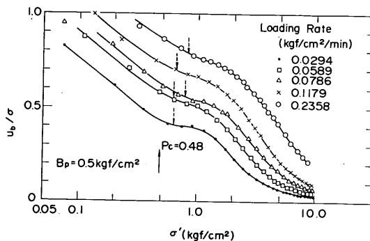
図-4.26 定載荷速度圧密試験の間隙水圧比と有効応力の関係(本牧再圧密試料)
