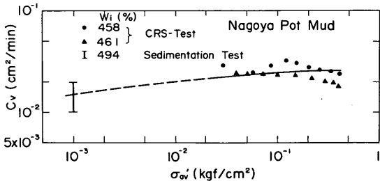
図-6.17 沈降試験及び定ひずみ速度圧密試験にもとづく圧密係数と有効応力の関係 (名古屋港泥土)
