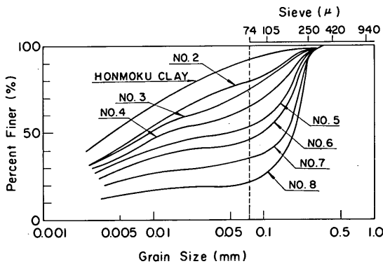
図-8.7 各試料の粒度分布
