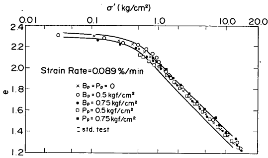
図 - 4.5 a 予圧密とバックプレッシャーの影響 (CRS-Test, 本牧再圧密試料)
