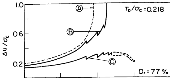
図一 9.1 繰返し載荷強度に及ぼす部分排水の影響 (Lee-Pocht, 1975)
