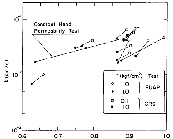
図-9.21 3種類の試験による k と初期間隙比の関係(PUAP:加圧透水試験, CRS:定ひずみ速度圧密試験)
