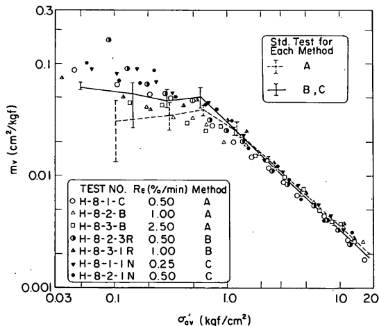
図一8.23 a m_v 特性とひずみ速度 (Mix. No. 8 試料)
