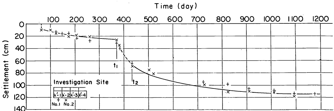
図一 8.33 沈下量の実測値と計算値
