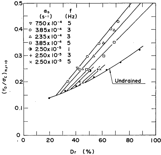
図-9.13a N_i=10 で液状化を生ずる応力比と相対密度の関係
