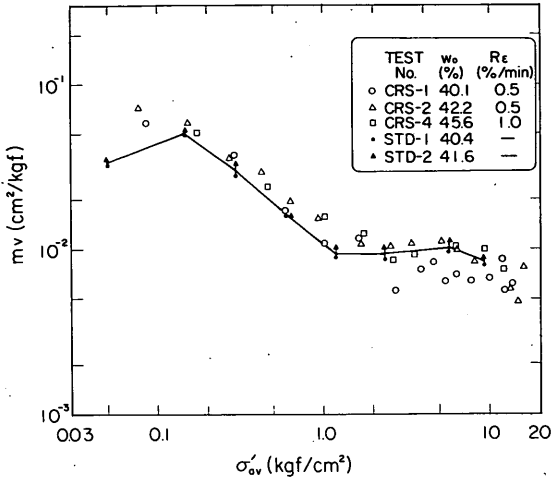
図一 8.32 a 定ひずみ速度圧密試験及び標準圧密試験による m_v と平均圧密応力の関係
