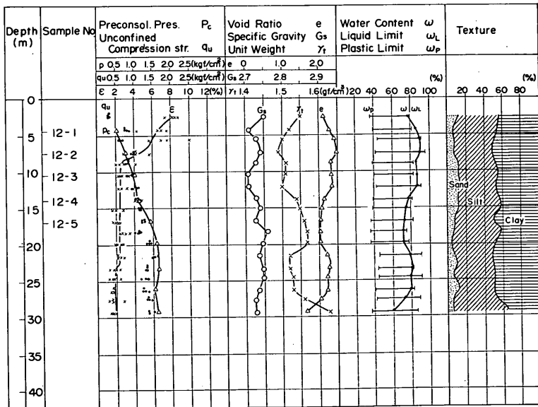
図-4.4 b 大黒町自然試料 (No 12) の土性図
