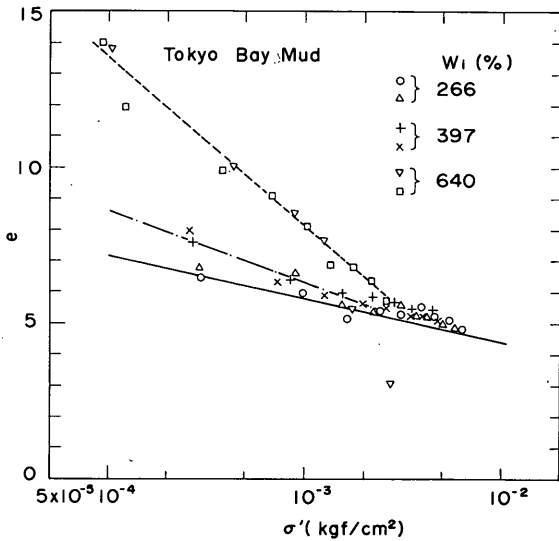
図-6.5 b 沈降試験より定めた e \sim \log \sigma' 関係 (東京湾泥土)
