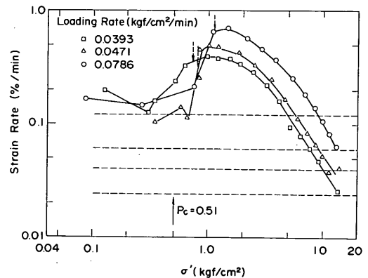
図-4.22 定載荷速度圧密試験のひずみ速度の有効応力に対する変化と載荷速度(錦海自然試料No.46-1)
