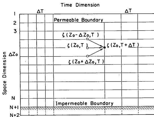
図一7.6 差分間隔
