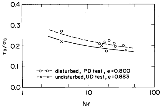
図-9.27 排水条件が異なる場合の \tau_D/\sigma_c \sim N_e 関係 ( \bar{\alpha} = 0 の場合と \bar{\alpha} = 1.85 \times 10^{-6} の場合)
