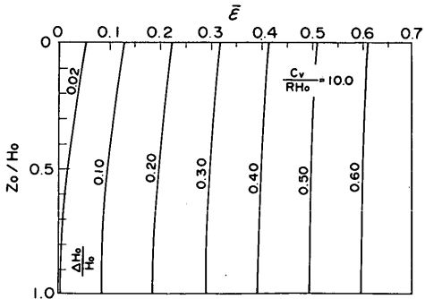
図-3.4 c 平均ひずみの変化に対する供試体内のひずみ分布 ( c_v/(RH_0) = 10 の場合)
