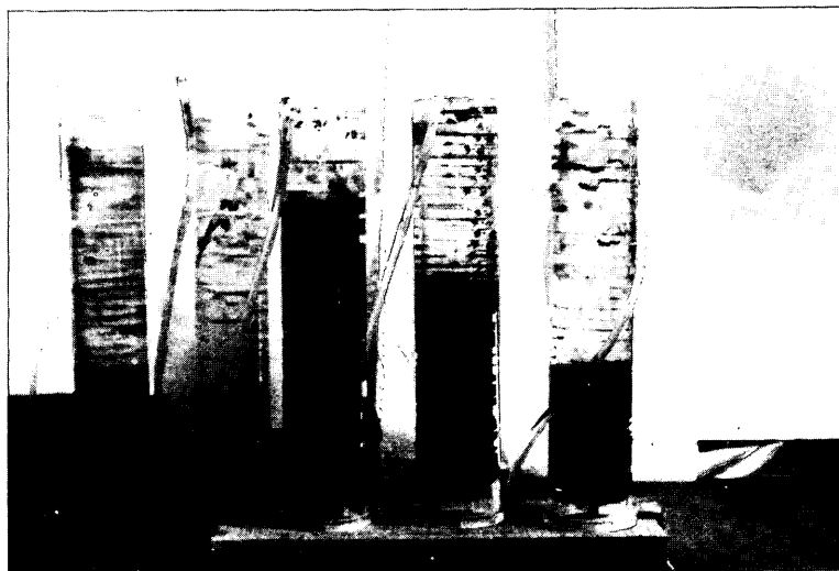
写真-6.1 二重円筒型沈降試験装置
