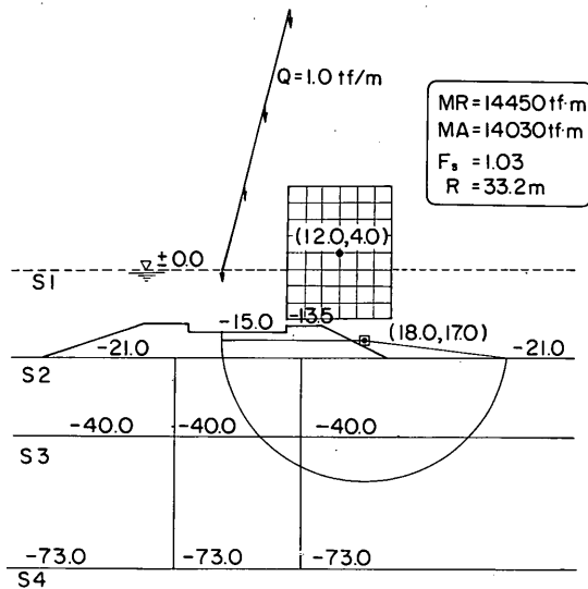
図-8.30 安定計算結果(波圧時)
