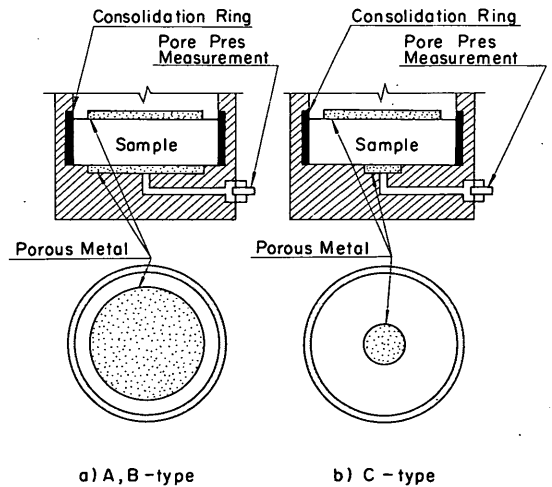
図-8.11 試験方法の分類
