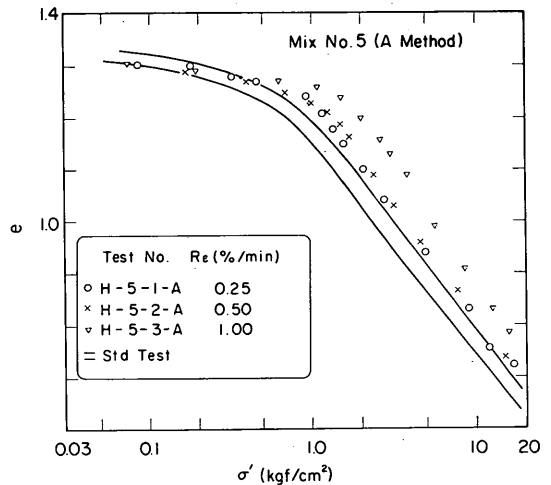
図一 8.19 e \sim \log \sigma' 関係に及ぼすひずみ速度の影響 (Mix. No. 5 試料, A法)
