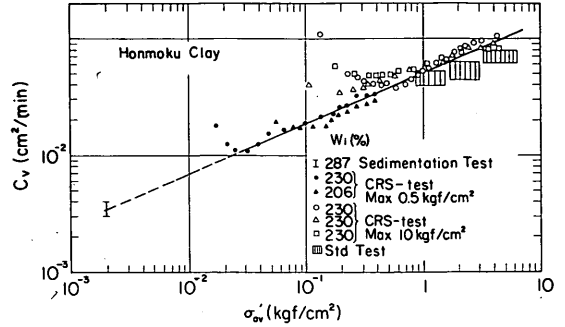
図-6.14 広範囲の応力領域における圧密係数と有効応力の関係(本牧粘土)
