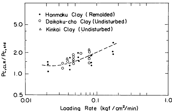
図-4.14 圧密降伏応力と載荷速度
