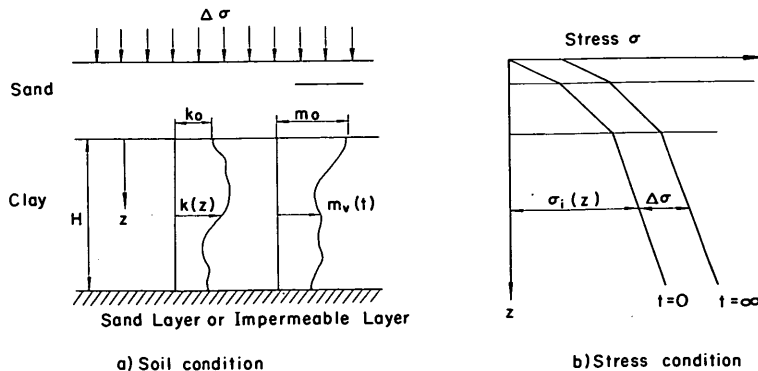
図-8.2 不均質地盤の圧密
