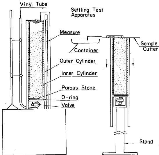
図-6.2 沈降試験装置模式図
