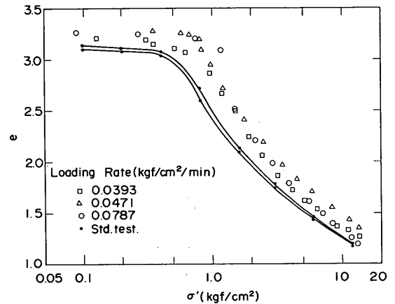
図 - 4.12 b e \sim \log \sigma' 曲線に及ぼす定載荷速度圧密試験の載荷速度の影響 (錦海自然試料 No. 46-1, B_p = 1.1 \text{ kgf/cm}^2 )
