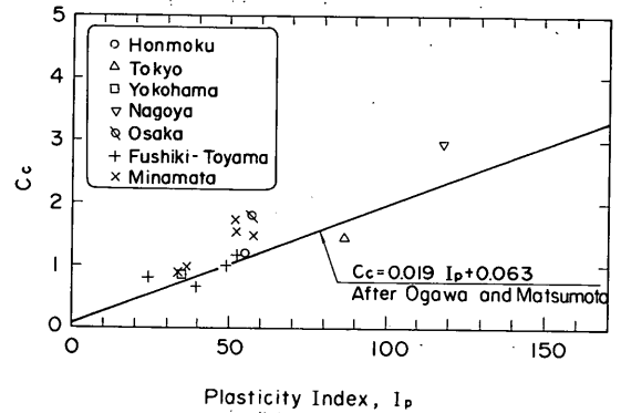
図-6.22 圧縮指数 C_c と塑性指数の関係
