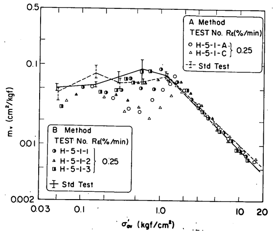
図-8.17 a m_v \sim \sigma'_{ov} 関係に及ぼす試験法の影響 (Mix.No.5 試料)
