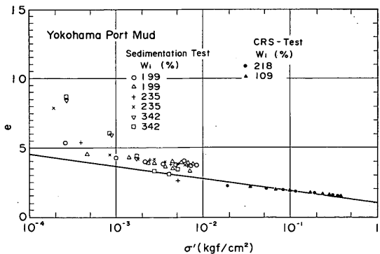
図-6.9 沈降試験及び定ひずみ速度圧密試験にもとづく e \sim \log \sigma' 関係 (横浜港泥土)
