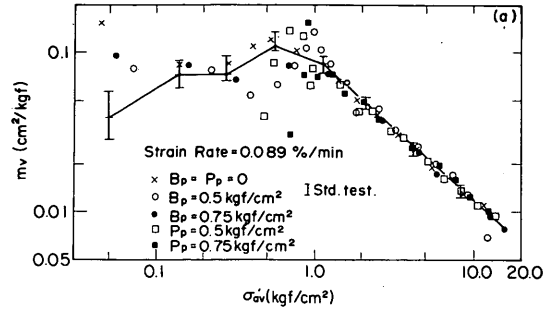
図 - 4.6 a 予圧密とバックプレッシャーの影響 (CRS-Test, 本牧再圧密試料)
