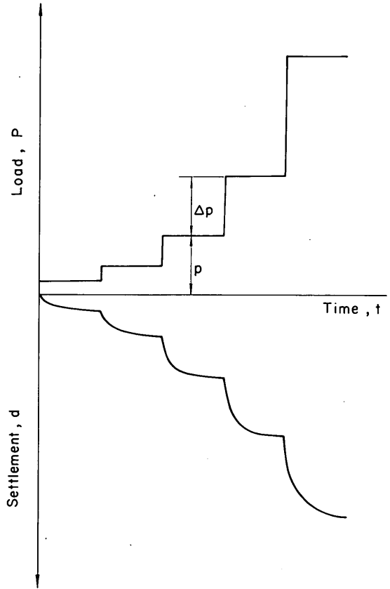
図-2.5 標準圧密試験の荷重形式の模式図
