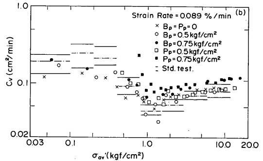
図 - 4.6 b 予圧密とバックプレッシャーの影響 (CRS-Test, 本牧再圧密試料)
