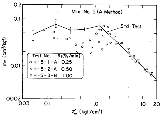
図-8.21 a m_v 特性とひずみ速度 (Mix.No.5 試料)
