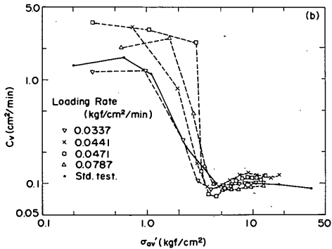
図-4.19 圧密定数に及ぼす定載荷速度圧密試験の載荷速度の影響(大黒町自然試料No.6-7, B_p = 3.0 \text{ kgf/cm}^2 )
