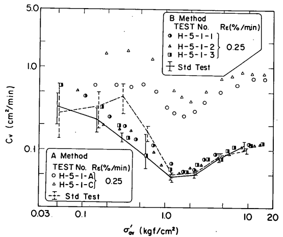
図-8.17 b c_v \sim \sigma'_{ov} 関係に及ぼす試験法の影響 (Mix.No.5 試料)
