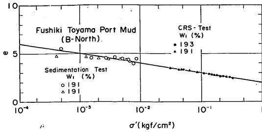
図-6.12 b 沈降試験及び定ひずみ速度圧密試験にもとづく e \sim \log \sigma' 関係 (伏木富山港泥土 B-North)
