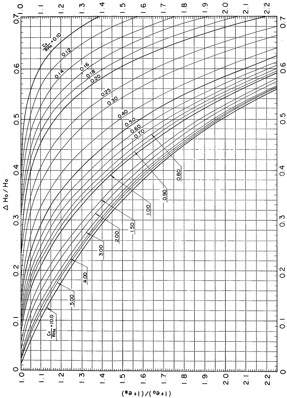
図-3.6 a 下端面の圧密比の平均比の平均比に対する変化
