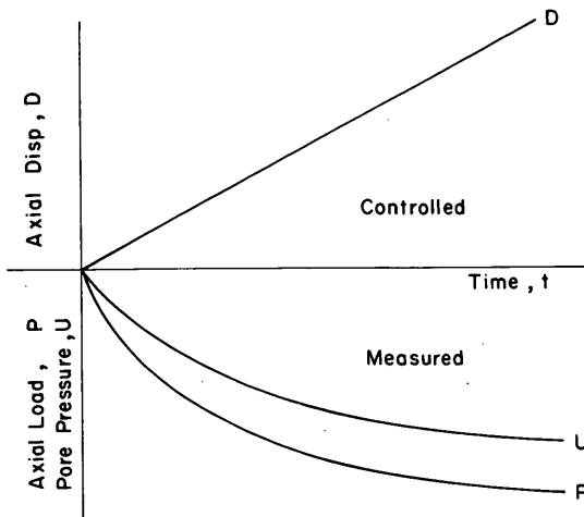
図-2.6 定ひずみ速度圧密試験の模式図
