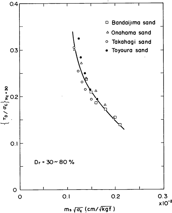
図-9.16 b N_t = 20 で液状化を生ずる応力比と m_s \sqrt{\sigma_c} の関係
