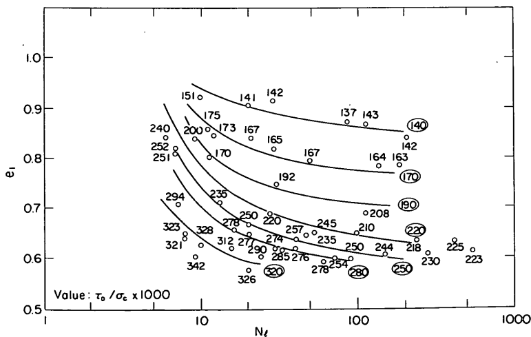
図一9.10 e_i \sim N_t \sim \tau_D/\sigma_c 関係(完全非排水条件, \alpha_b=0 )
