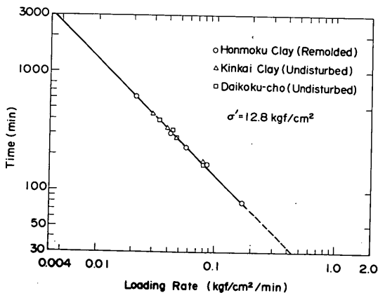
図-4.29 載荷速度と試験所要時間
