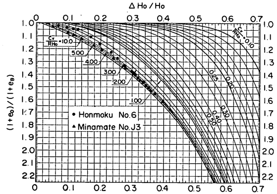
図-5.8 (1+e_0)/(1+e_B) \sim \Delta H_0/H_0 プロット例
