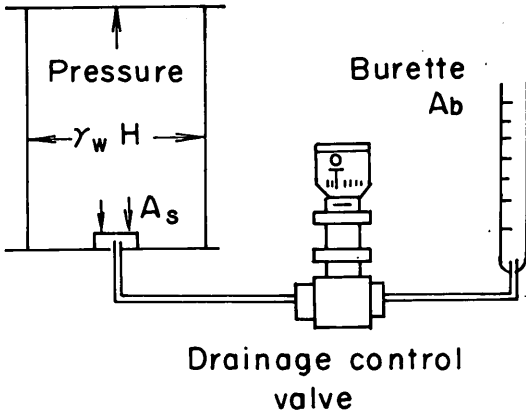
図一 9.4 排水制御系模式図
