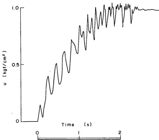
図一9.9 a 部分排水条件のもとでの液状化試験記録例(万代島砂, e_i=0.781 , \sigma_c=1.0 \text{ kgf/cm}^2 , \alpha_b=3.85 \times 10^{-4} \text{ s}^{-1} , f=5 \text{ Hz} )
