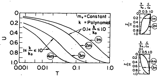
図-8.3 各条件に対するU-T曲線 (Schiffman-Gibson, 1964)
