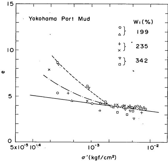
図-6.5 c 沈降試験より定めた e \sim \log \sigma' 関係 (横浜港泥)
