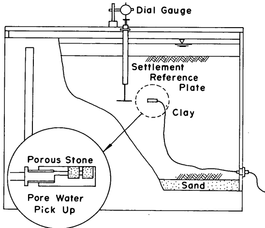
図一7.1 自重圧密実験槽模式図
