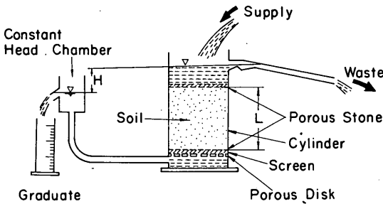
図一 9.5 透水試験模式図
