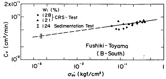
図-6.19 a 沈降試験及び定ひずみ速度圧密試験にもとづく圧密係数を有効応力の関係 (伏木富山港泥土 B-South)
