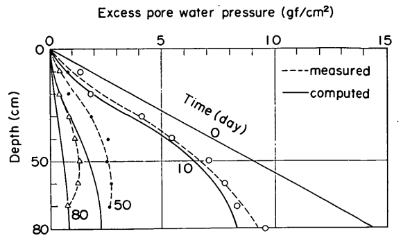
図-7.9 自重圧密過程における過剰間隙水圧分布の経時変化の実測値と理論値の比較 (本牧粘土)
