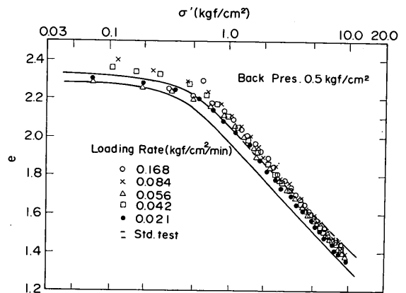
図-4.10b e \sim \log \sigma' 曲線に及ぼす載荷速度の影響(CLR-Test)
