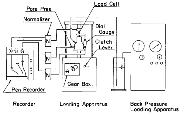
図-8.10 定ひずみ速度圧密試験装置の構成図
