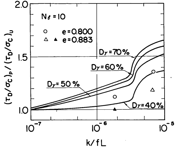
図-9.29 液状化強度比と排水効果係数の関係の比較例
