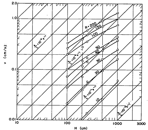
図一 9.6 v, H 及び k/L の関係
