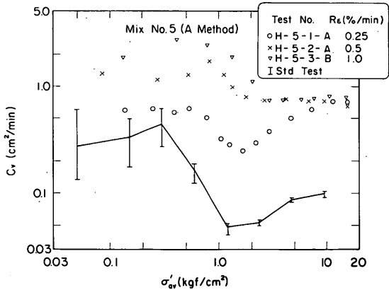
図-8.21 b c_v 特性とひずみ速度 (Mix.No. 5 試料)
