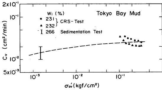
図-6.15 沈降試験及び定ひずみ速度圧密試験にもとづく圧密係数と有効応力の関係 (東京湾泥土)
