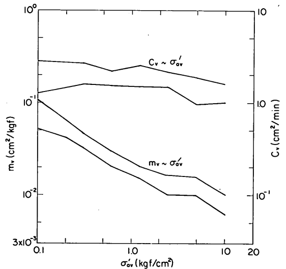
図-8.28 c 標準圧密試験による m_v と c_v
