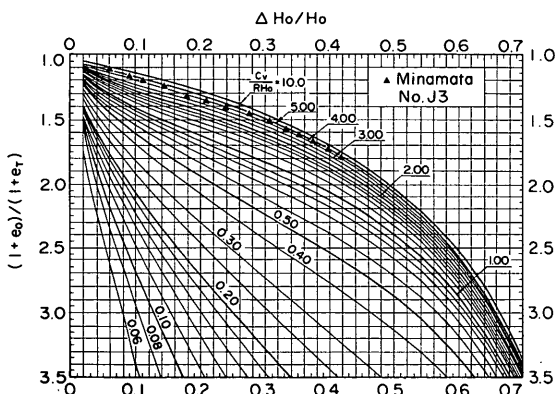
図-5.7 (1+e_0)/(1+e_T) \sim \Delta H_0/H_0 プロット例
