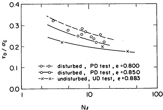
図-9.28 排水条件が異なる場合の \tau_D/\sigma_c \sim N_e 関係 ( \bar{\alpha} = 0 の場合と \bar{\alpha} = 7.0 \times 10^{-6} の場合)
