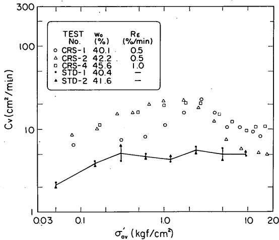
図一 8.32 b 定ひずみ速度圧密試験及び標準圧密試験による c_v と平均圧密応力の関係
