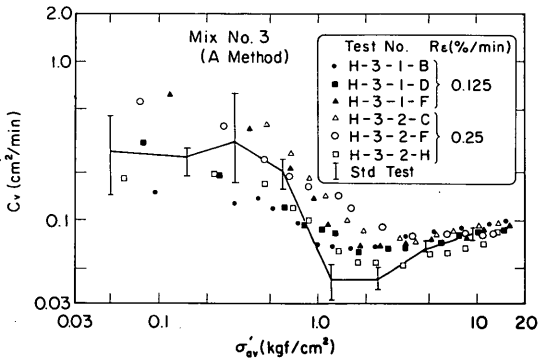
図-8.16 b c_v \sim \sigma'_{ov} 関係 (Mix.No.3 試料, A法)
