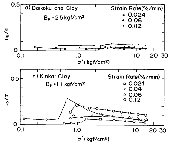
図-4.24 定ひずみ速度圧密試験の間隙水圧比と有効応力の関係(大黒町自然試料及び錦海自然試料)
