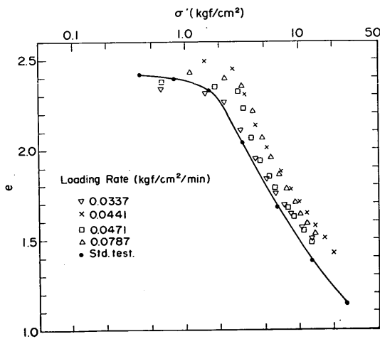
図 - 4.11 b e \sim \log \sigma' 曲線に及ぼす定載荷速度圧密試験の載荷速度の影響 (大黒町自然試料 No. 6-7, B_p = 3.0 \text{ kgf/cm}^2 )
