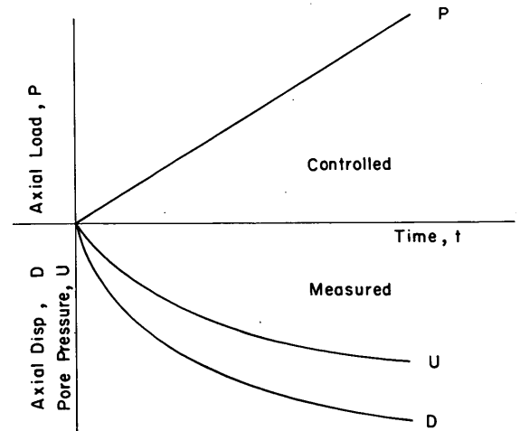
図-2.7 定載荷速度圧密試験の模式図
