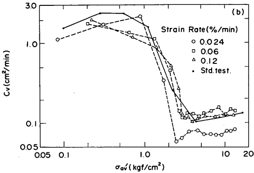
図-4.17 圧密定数に及ぼす定ひずみ速度圧密試験のひずみ速度の影響(大黒町試料, No.6-1, B_p = 2.5 \text{ kgf/cm}^2 )
