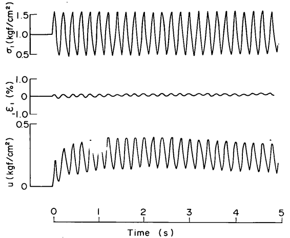
図一9.9 b 部分排水条件のもとでの液状化試験の記録例(万代島砂, e_i=0.771 , \sigma_c=1.0 \text{ kgf/cm}^2 , \alpha_b=3.84 \times 10^{-4} \text{ s}^{-1} , f=5 \text{ Hz} )
