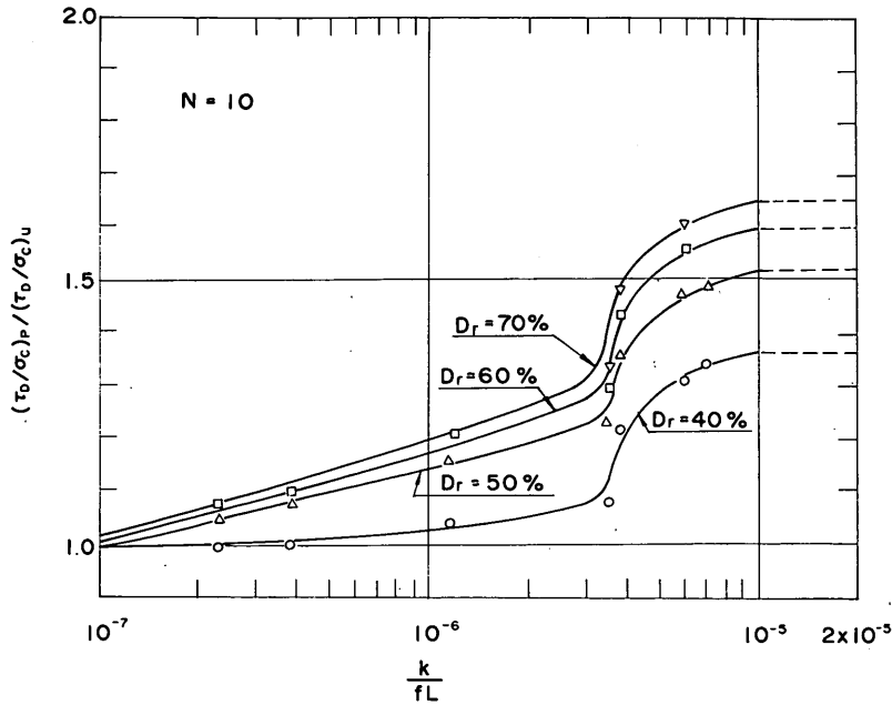
図一 9.14 a 液状化強度比と k/(fL) の関係 ( N_t = 10 )
