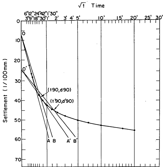
図一 8.6 圧密定数決定のための \sqrt{t} 法適用例 (小林ら, 1974)
