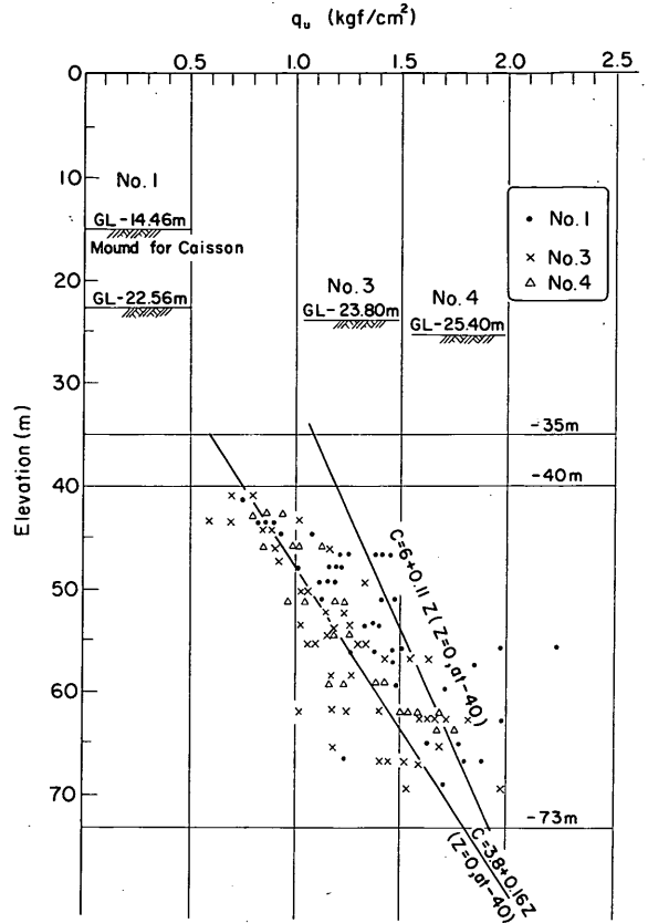
図-8.28 b q_u の深さ分布
