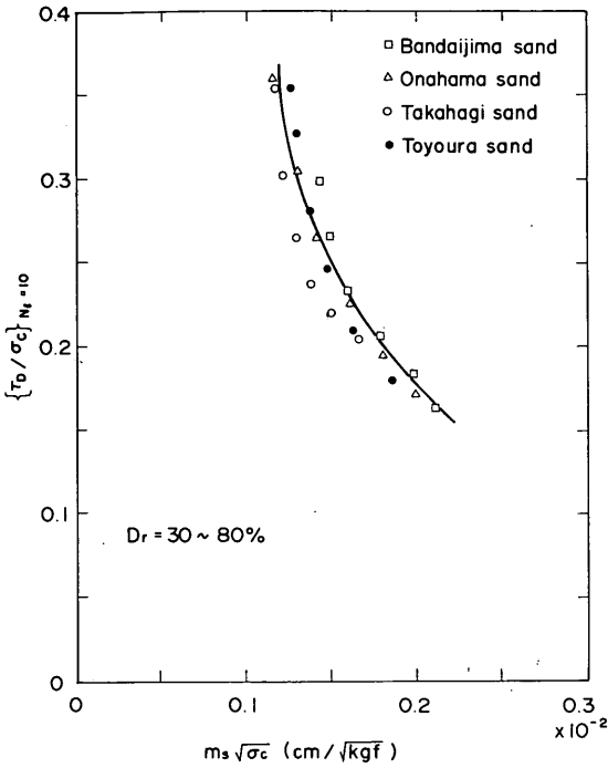
図-9.16 a N_t = 10 で液状化を生ずる応力比と m_s \sqrt{\sigma_c} の関係
