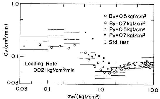
図 - 4.6 d 予圧密とバックプレッシャーの影響 (CLR-Test, 本牧再圧密試料)
