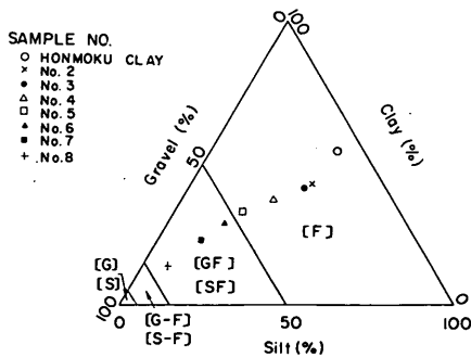
図-8.8 各試料の分類特性
