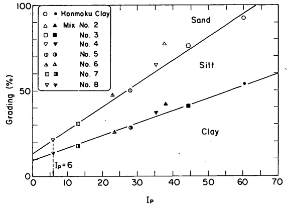
図-8.9 塑性指数 I_p と粘土分含有量の関係
