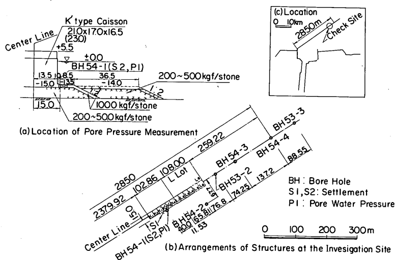
図-8.27 構造物位置図及び土質調査実施地点
