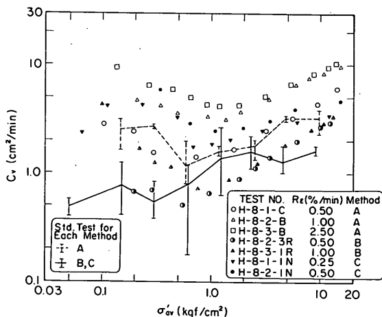
図一8.23 b c_v 特性とひずみ速度 (Mix. No. 8 試料)
