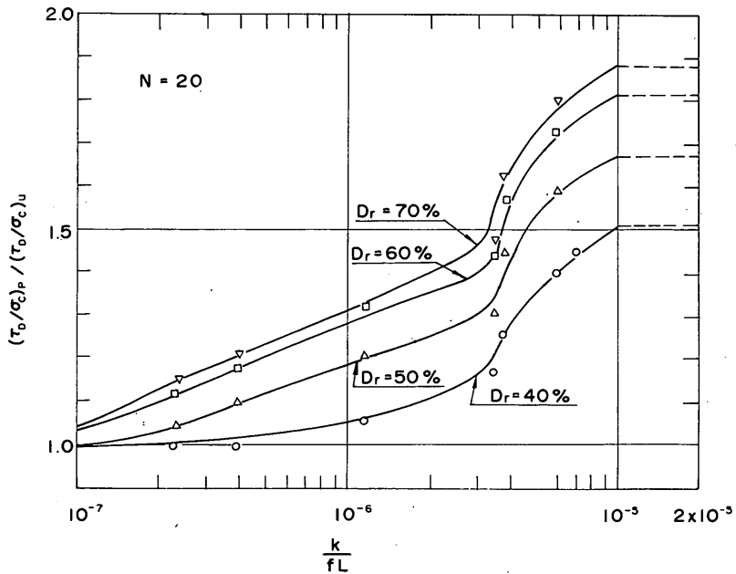
図一 9.14 b 液状化強度比と k/(fL) の関係 ( N_t = 20 )
