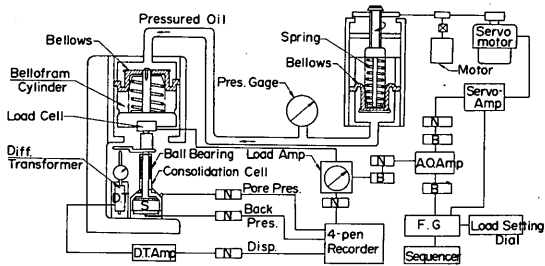
図-4.2 定載荷速度試験装置ブロック図
