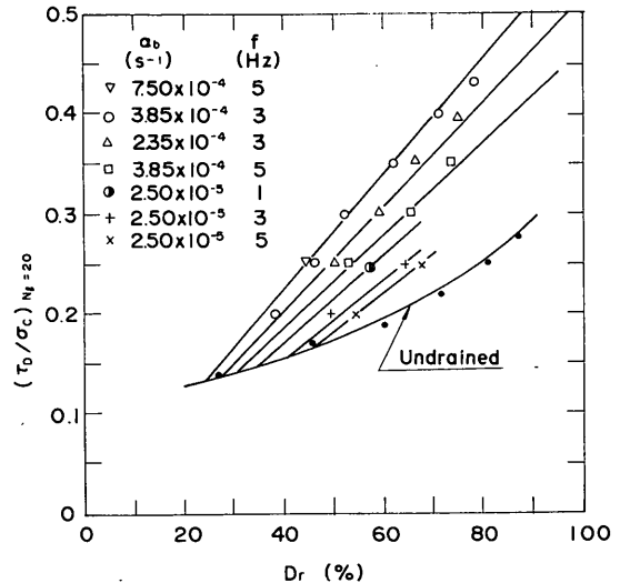
図-9.13b N_i=20 で液状化を生ずる応力比と相対密度の関係
