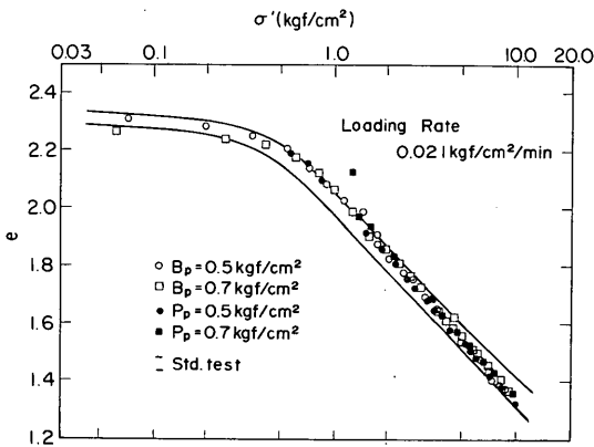
図 - 4.5 b 予圧密とバックプレッシャーの影響 (CLR-Test, 本牧再圧密試料)
