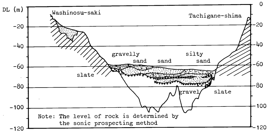
図-9.25b 土質断面図
