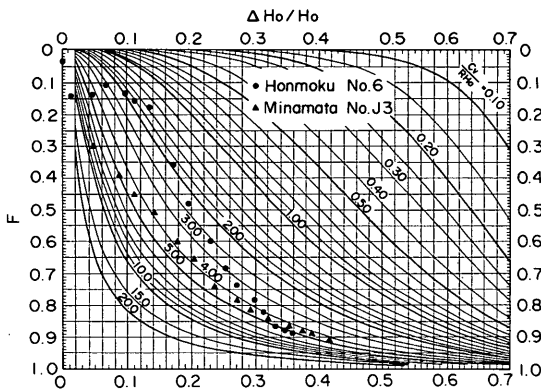
図-5.6 F \sim \Delta H_0/H_0 プロット例
