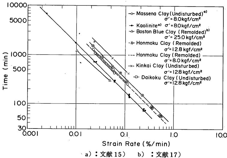
図-4.28 特定有効応力に到達するに要する時間とひずみ速度 (定ひずみ速度圧密試験)
