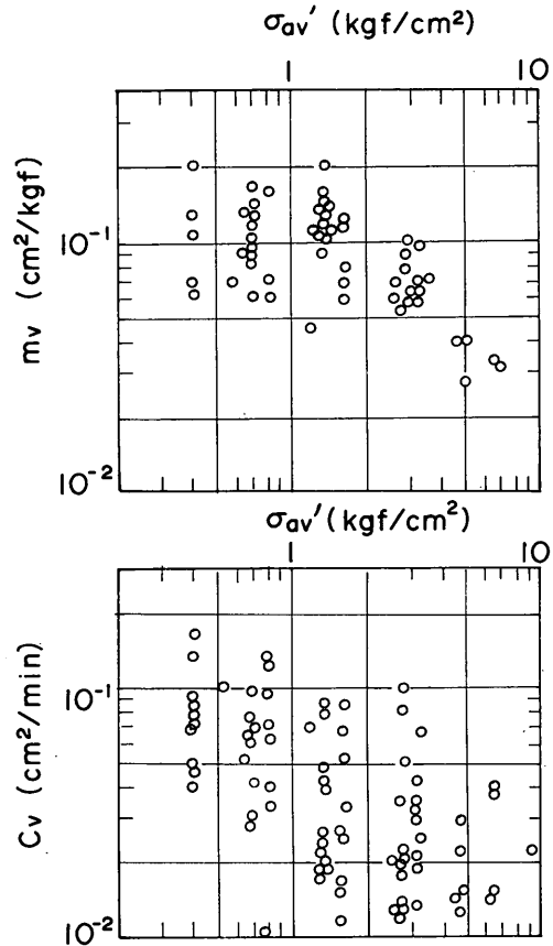
図-5.2 浚渫前の粘土土料の圧密特性 (柳瀬, 1965)
