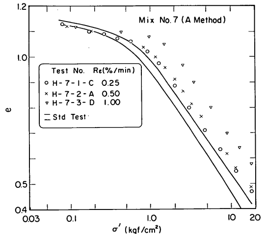
図一 8.20 e \sim \log \sigma' 関係に及ぼすひずみ速度の影響 (Mix. No. 7 試料, A法)
