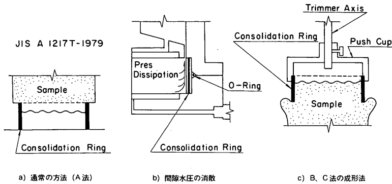
図-8.12 供試体の作成状況
