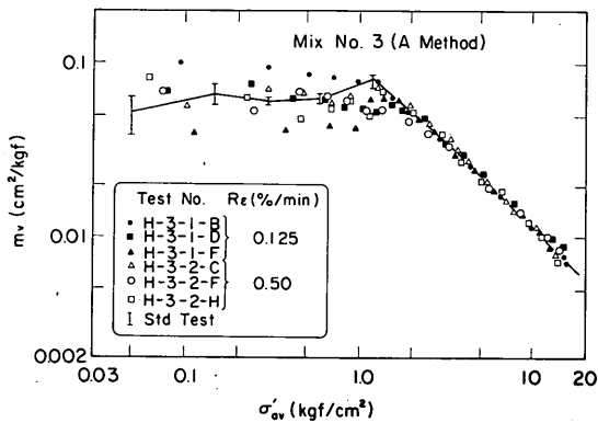
図-8.16 a m_v \sim \sigma'_{ov} 関係 (Mix.No.3 試料, A法)
