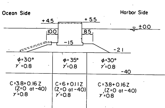
図-8.29 標準断面図
