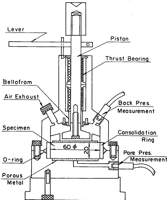
図-4.1 圧密容器
