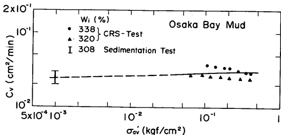
図-6.18 沈降試験及び定ひずみ速度圧密試験にもとづく圧密係数と有効応力の関係 (大阪湾泥土)
