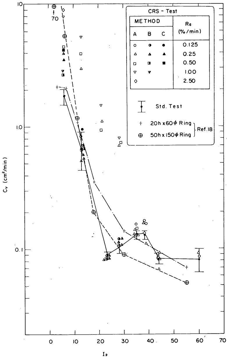
図一8.26 圧密係数 c_v と塑性指数 I_p の関係
