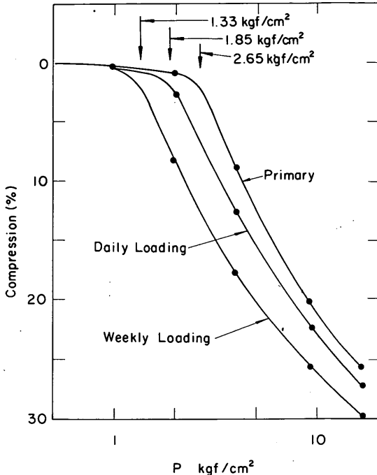
図-2.4 圧縮曲線に及ぼす荷重時間の影響 (Crawford, 1964)
