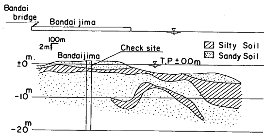
図-9.18 b 信濃川右岸の土質断面図 35)
