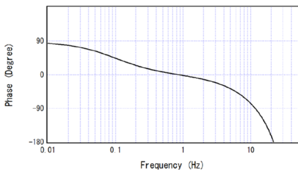
図-15 Dato1-100/Omni 型強震計の周波数特性
