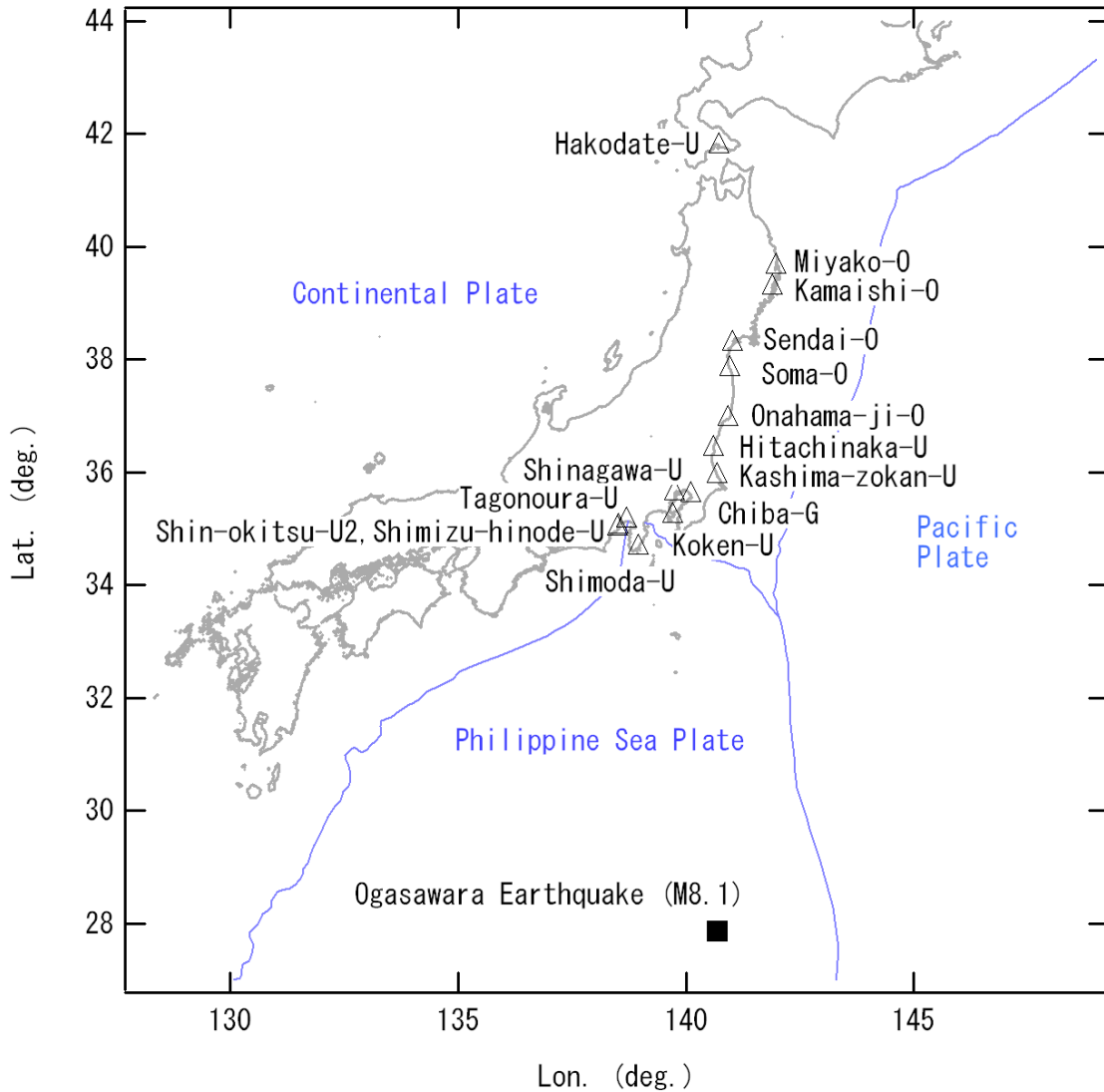
図-26 小笠原諸島西方沖の地震の震央 (■) と検討対象地点 (△)
