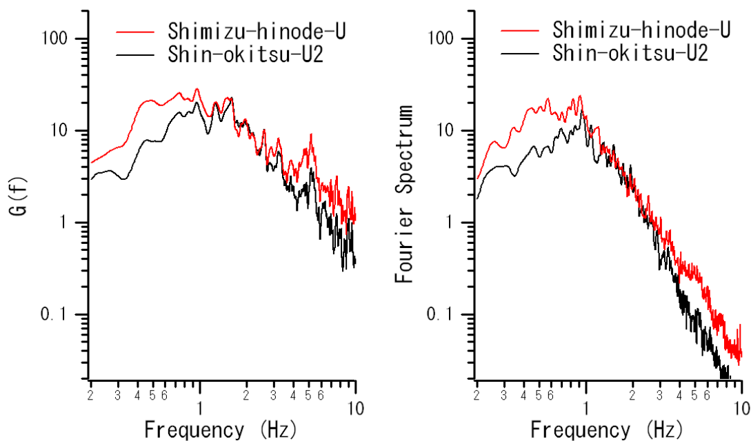
図-28 清水港の2地点におけるサイト増幅特性の比較(左)と観測された地震動のフーリエスペクトルの比較(右)
