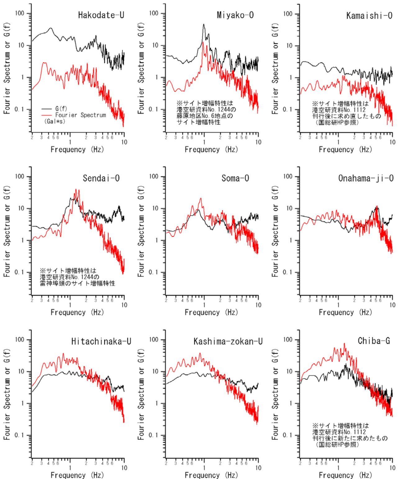
図-27 観測された地震動のフーリエスペクトルと当該地点のサイト増幅特性 G(f) との比較
