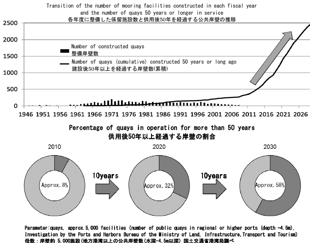
図 1.1 各年度に整備した係留施設数と供用後 50 年を経過する施設数の推移 1)
