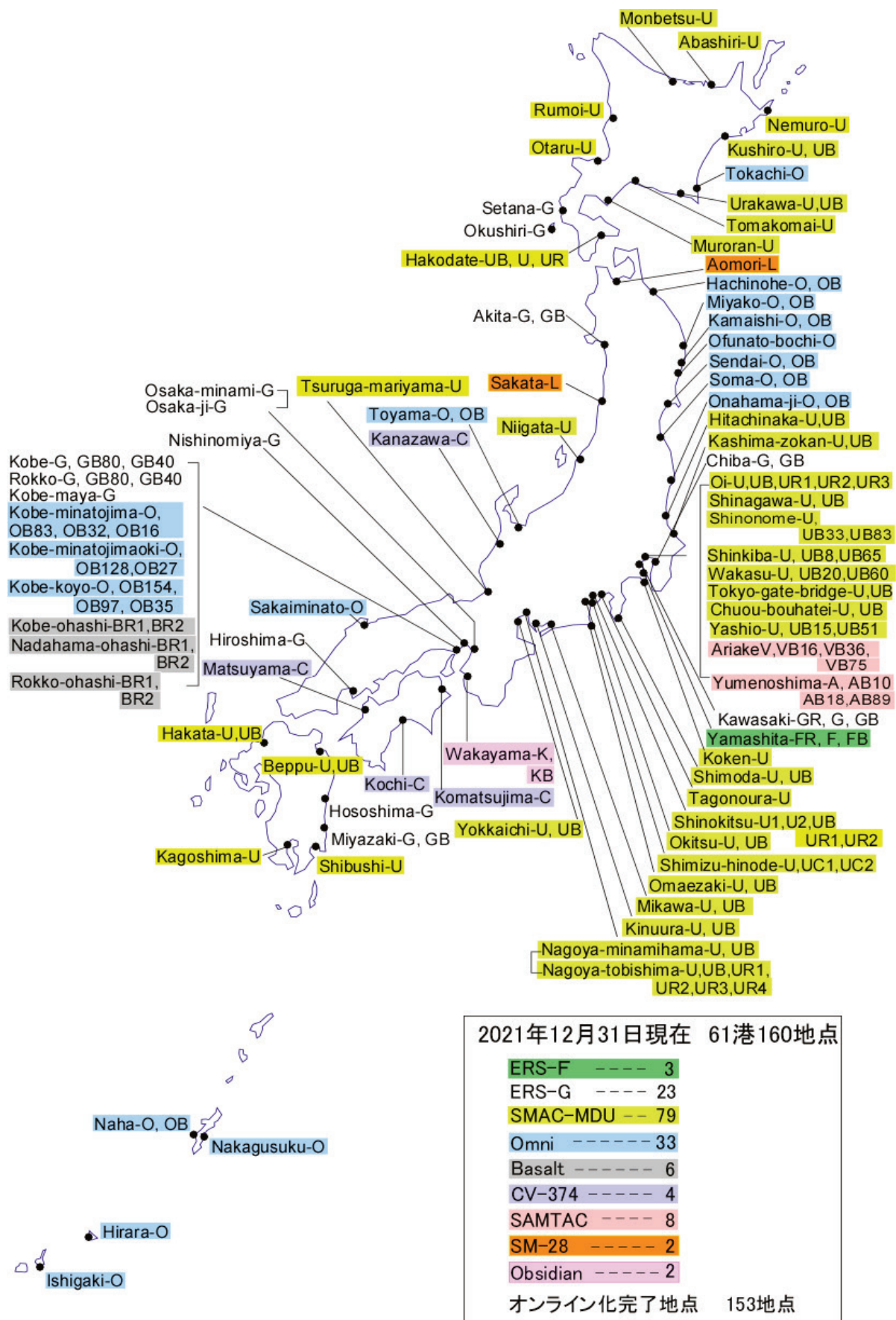
図-1 港湾地域強震観測網
