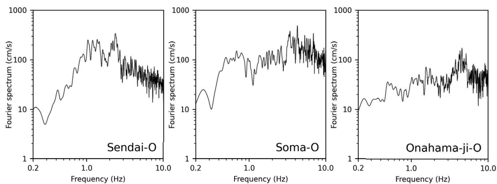
(c) 加速度フーリエスペクトル
