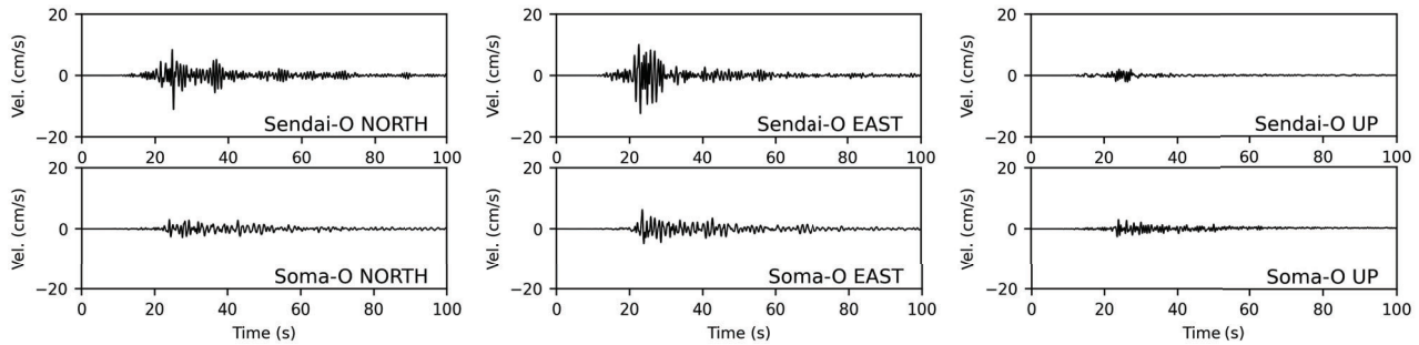
(b) 速度波形(0.2-2 Hz)
