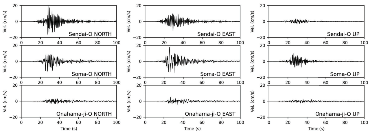
(b) 速度波形(0.2-2 Hz)
