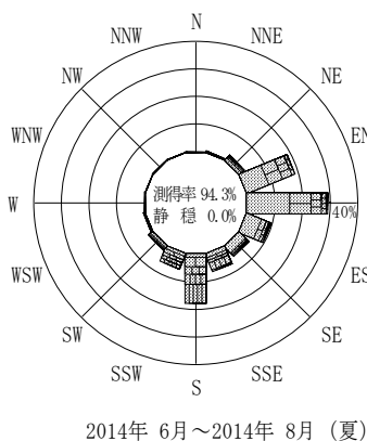
付図-B.2.76 高知西部沖 波高・波向別出現頻度図（連続観測）
