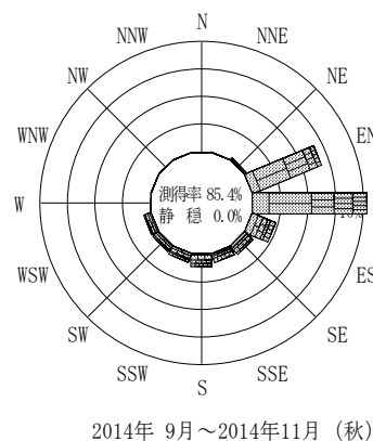
付図-B.2.76 高知西部沖 波高・波向別出現頻度図（連続観測）
