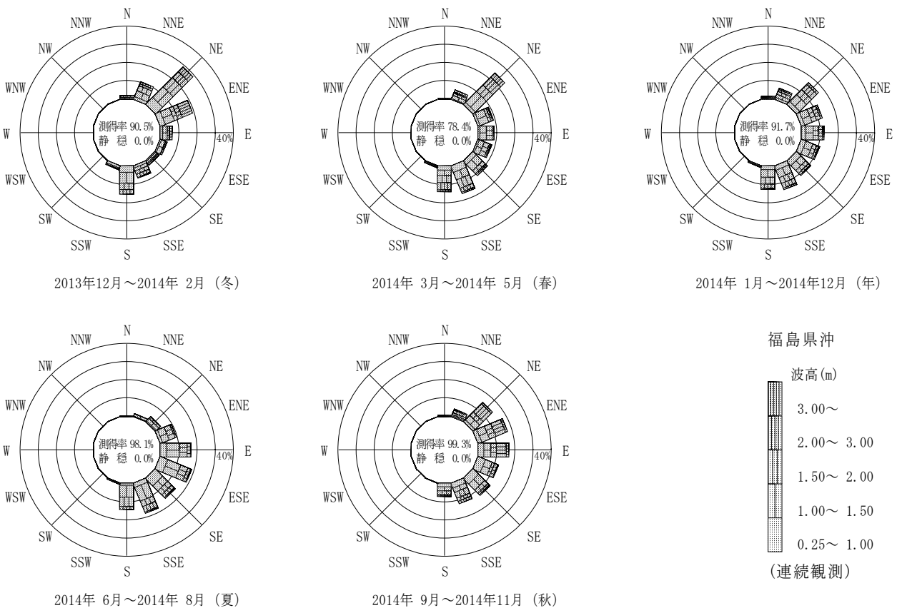
付図-B.2.70 福島県沖 波高・波向別出現頻度図（連続観測）
