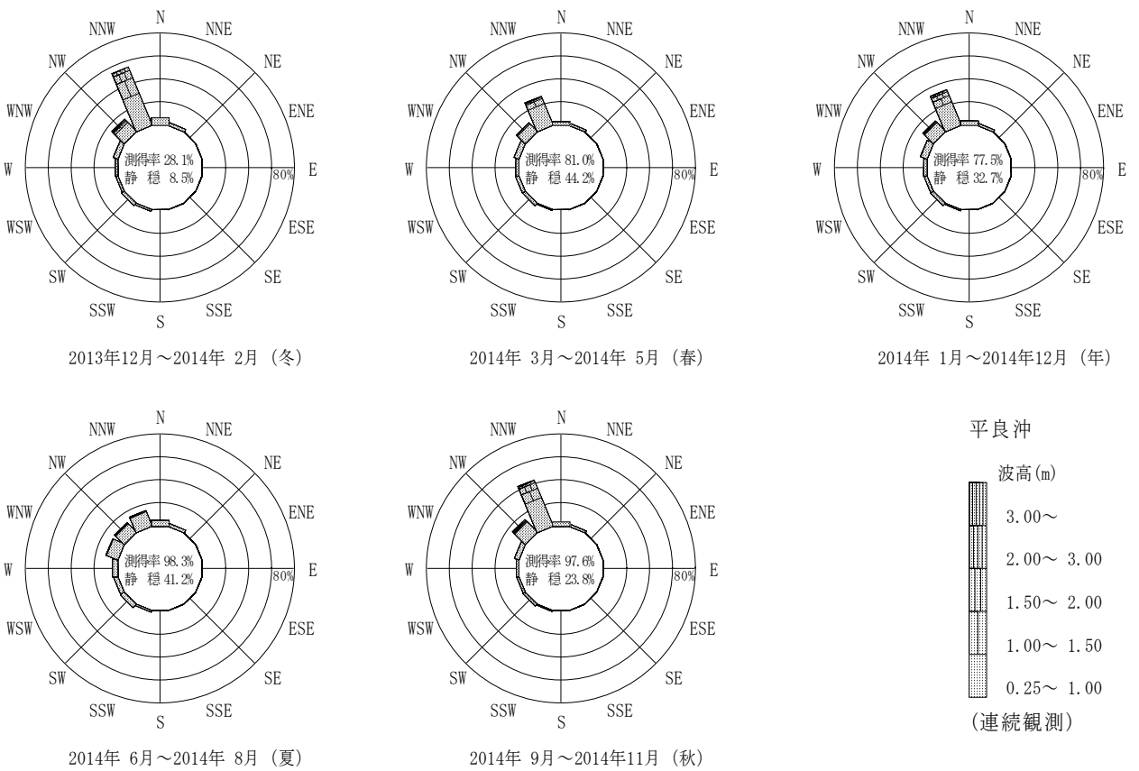
付図-B.2.59 平良沖 波高・波向別出現頻度図（連続観測）
