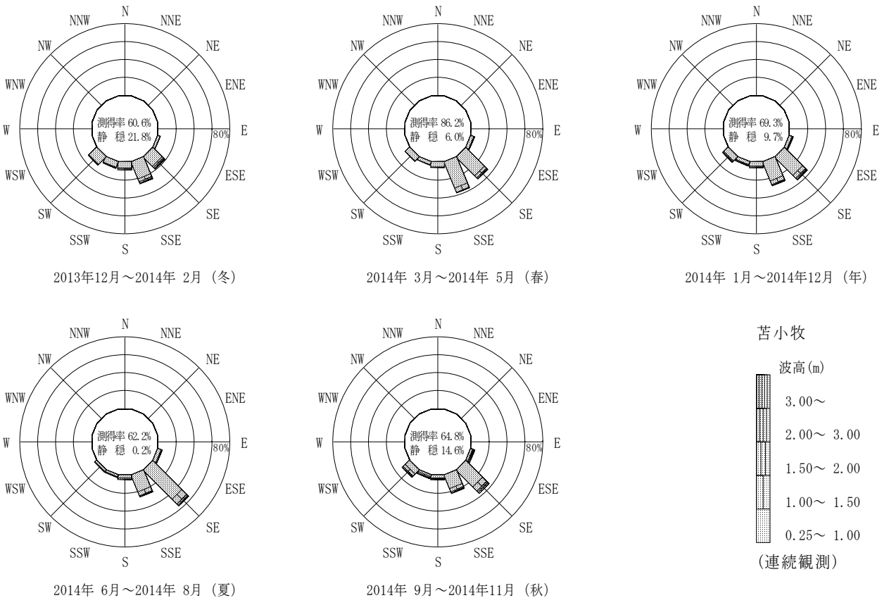
付図-B.2.30 苫小牧 波高・波向別出現頻度図（連続観測）
