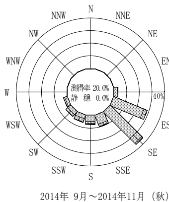
付図-B.2.44 下田 波高・波向別出現頻度図（連続観測）
