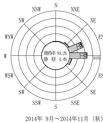
付図-B.2.35 釜石 波高・波向別出現頻度図（連続観測）
