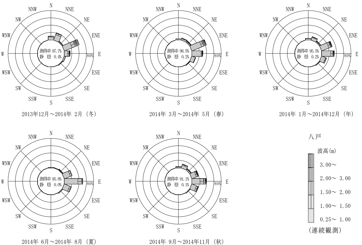
付図-B.2.32 八戸 波高・波向別出現頻度図（連続観測）
