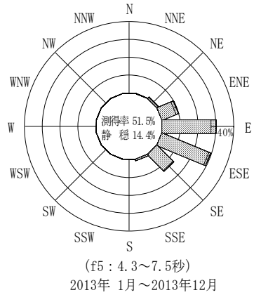
付図-B.3.38 相馬 波高・波向別出現頻度図 (連続観測, f2, f3, f4, f5, 全周期帯)
