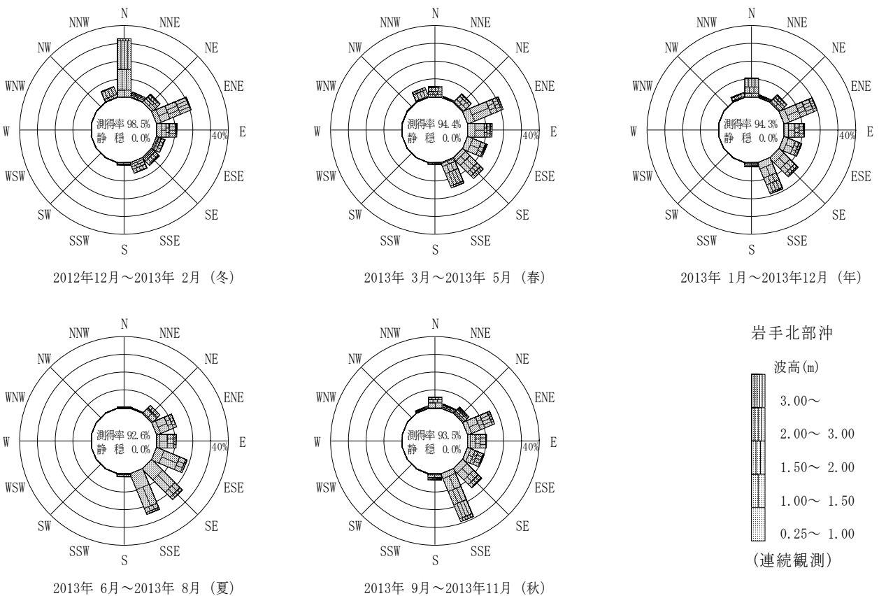
付図-B.2.65 岩手北部沖 波高・波向別出現頻度図（連続観測）
