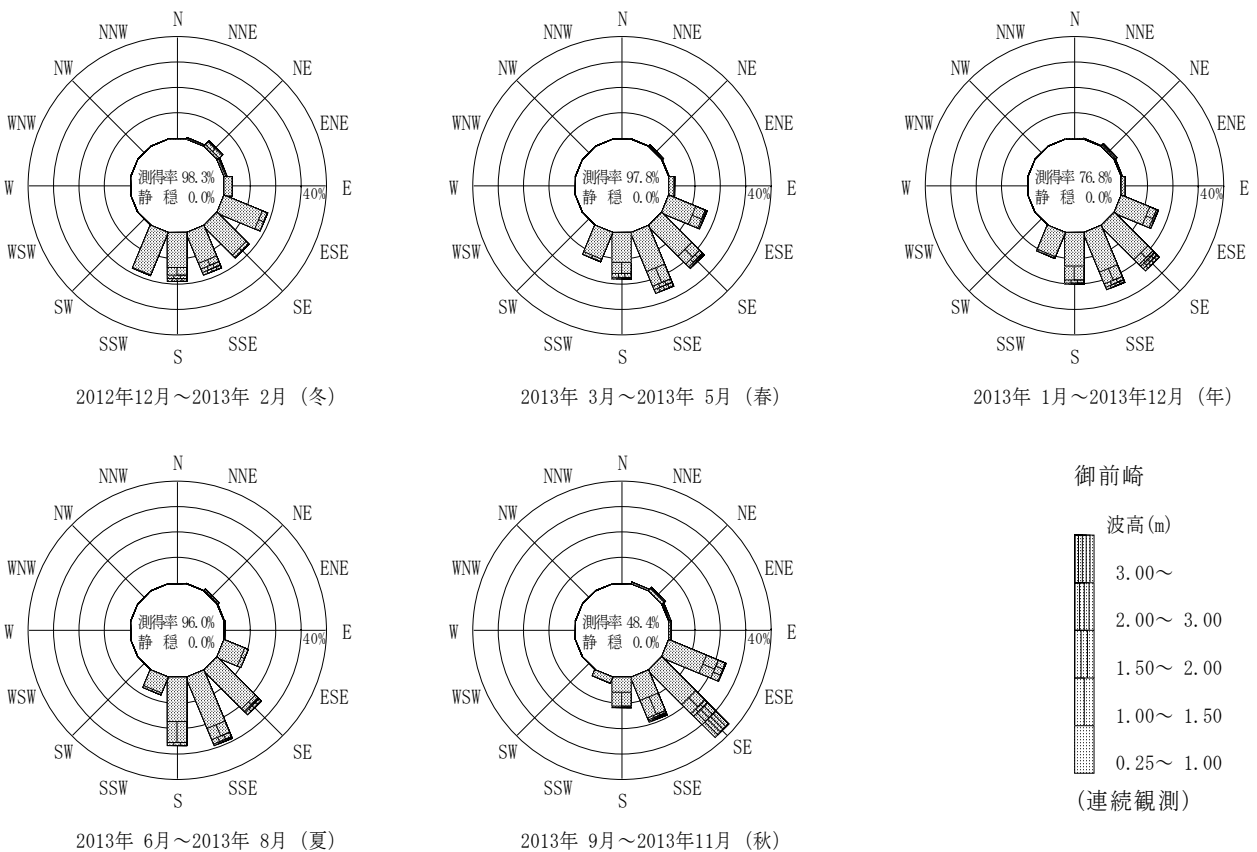
付図-B.2.46 御前崎 波高・波向別出現頻度図（連続観測）
