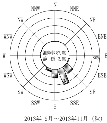
付図-B.2.52 高知 波高・波向別出現頻度図（連続観測）
