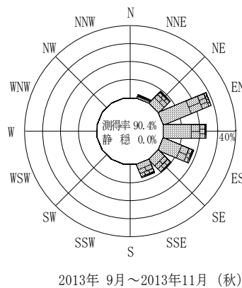
付図-B.2.38 相馬 波高・波向別出現頻度図（連続観測）
