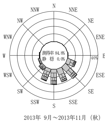
付図-A.2.28 釧路 波高・波向別出現頻度図
