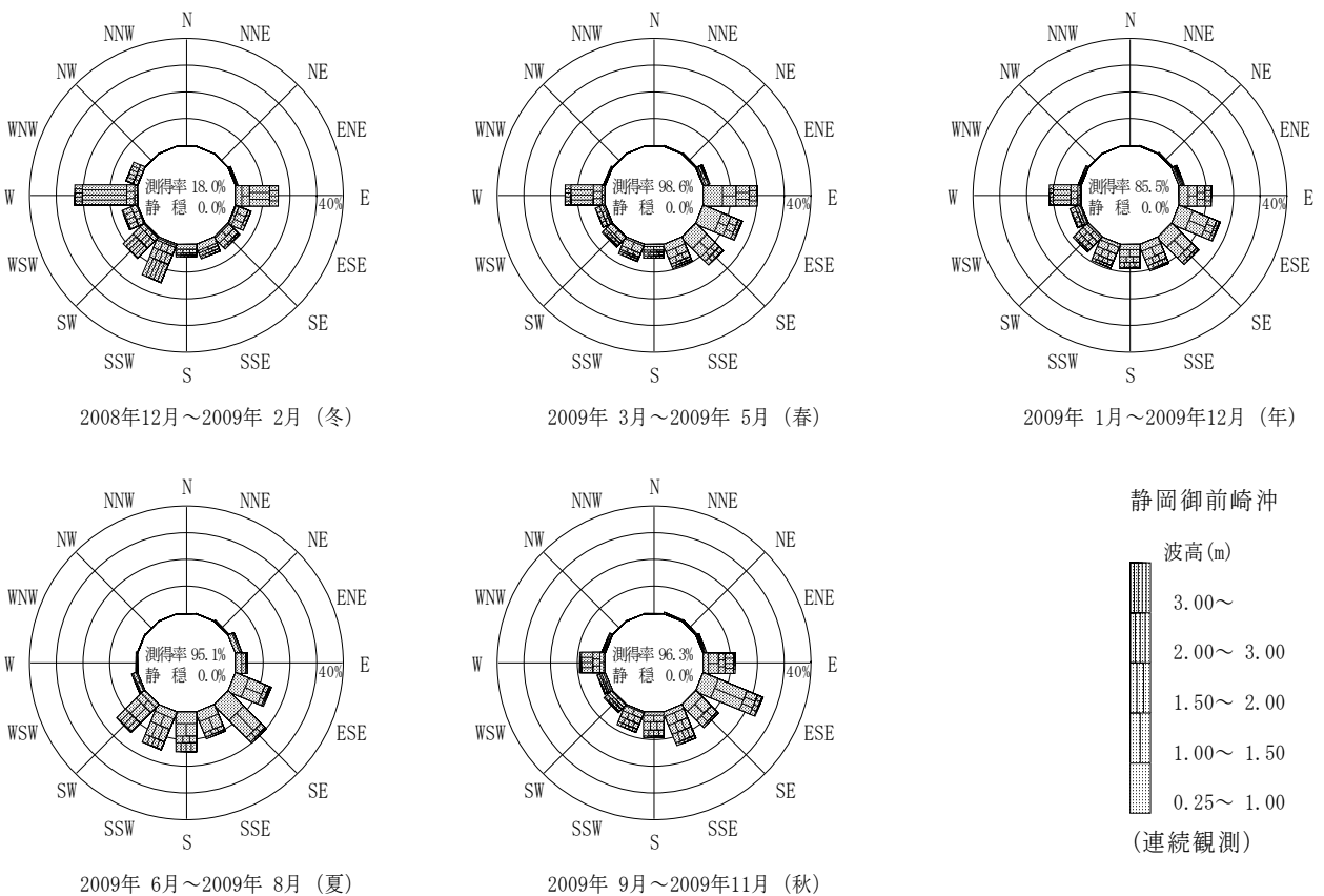
付図-B.2.69 静岡御前崎沖 波高・波向別出現頻度図 (連続観測)
