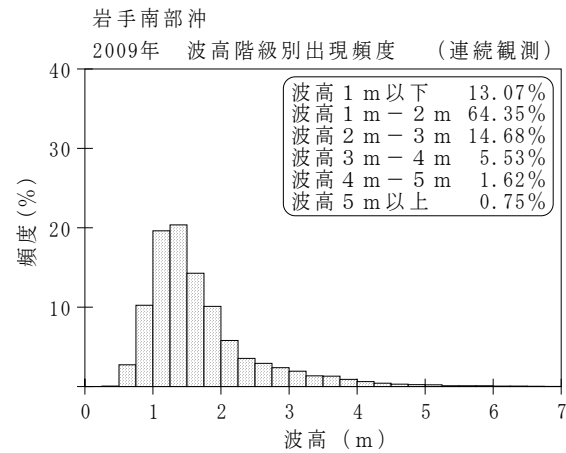
付図-B.1.65 岩手南部沖 波候特性図 (連続観測)
