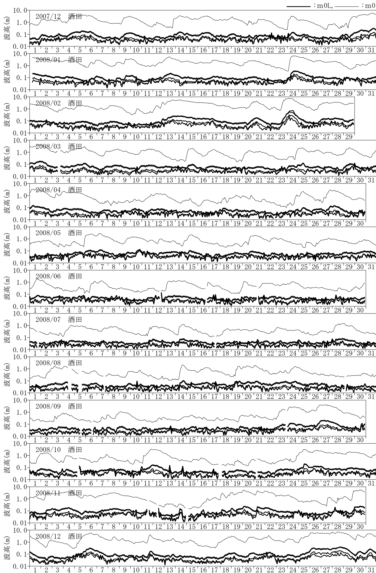
付図-C.1.7 長周期波高の経時変化図 (酒田)
