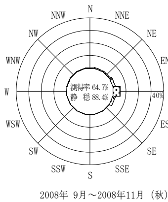
付図-B.2.55 苧田 波高・波向別出現頻度図（連続観測）
